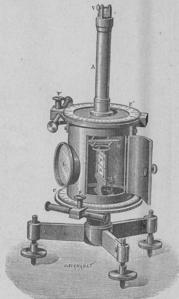
UNIFILAR PARA LAS VARIACIONES DE LA DECLINACIÓN
