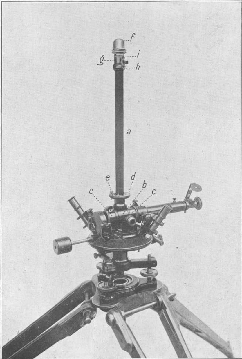
DECLINÓMETRO DE FIBRA
