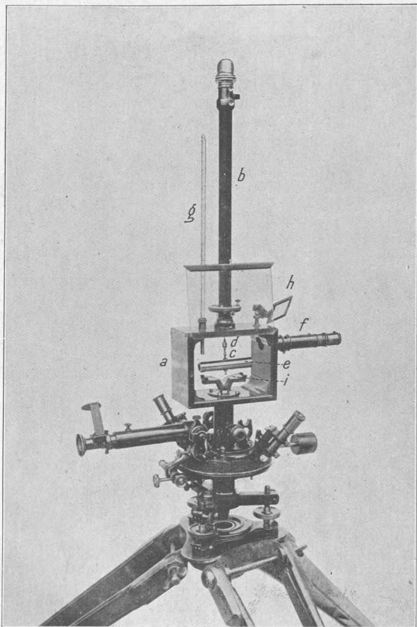
DISPOSICIÓN PARA OBSERVAR LAS OSCILACIONES EN LA MEDICIÓN DE LA COMPONENTE HORIZONTAL
