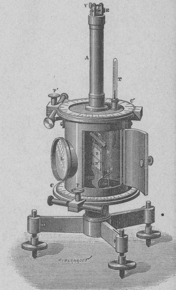
BIFILAR PARA LAS VARIACIONES DE LA COMPONENTE HORIZONTAL
