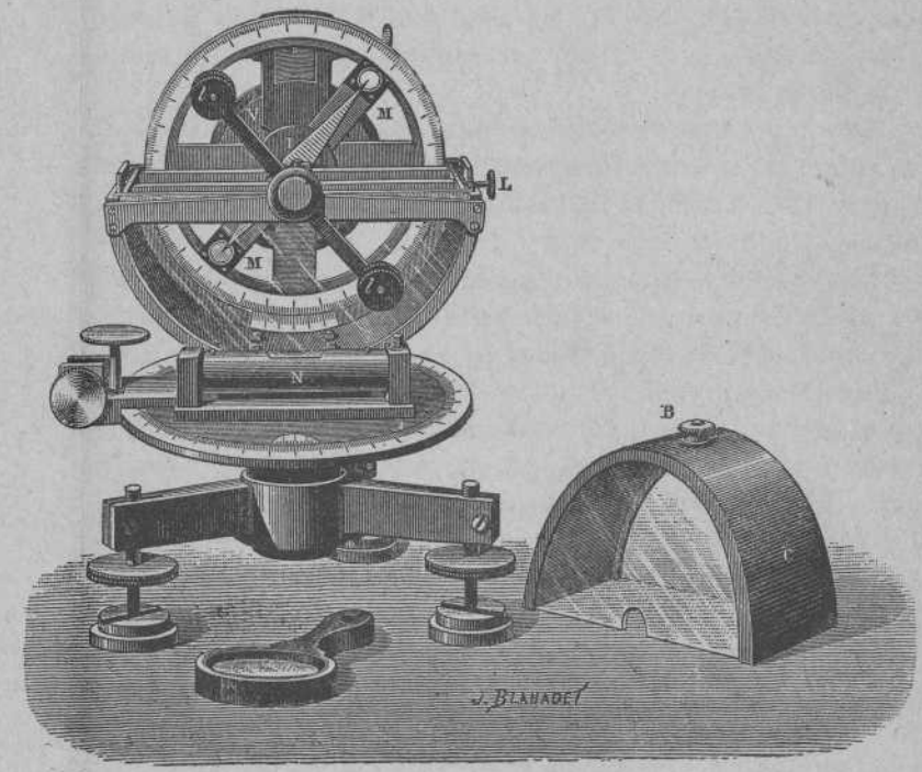
BRÚJULA DE INCLINACIÓN
