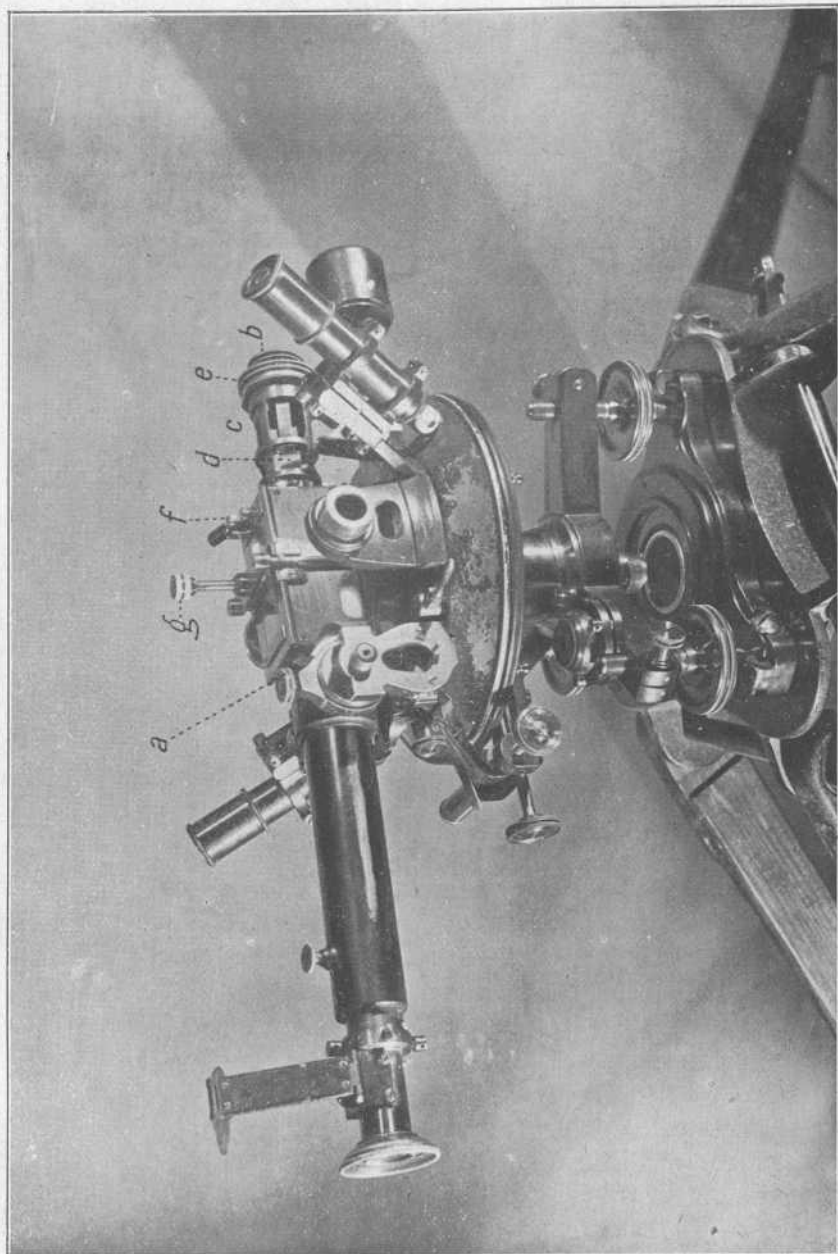
DECLINÓMETRO DE PIVOTE
