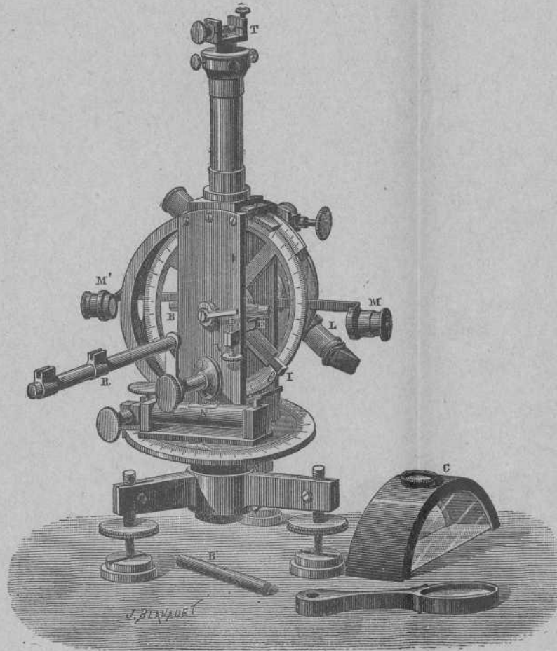
TEODOLITO MAGNÉTICO PARA MEDIR LA DECLINACIÓN Y COMPONENTE HORIZONTAL
