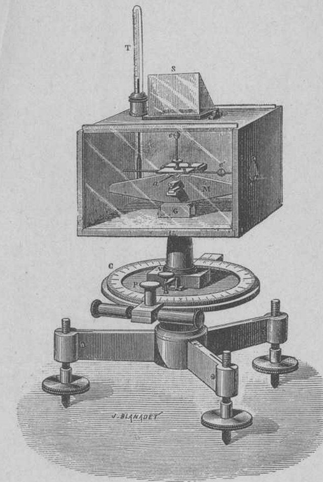
BALANZA PARA LAS VARIACIONES DE LA COMPONENTE VERTICAL
