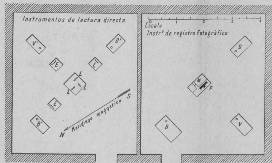
D, D' declinómetros. M. Cilindro registrador. L. Anteosjos V, V' Inclinómetros. B, B' bifilar. P, foco luminoso. E, Escalas para la lectura directa.
