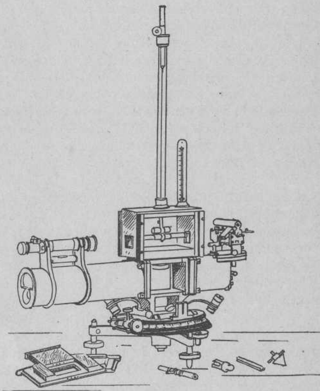
PARA DETERMINACIONES ABSOLUTAS DE LA DECLINACIÓN Y COMPONENTE HORIZONTAL
