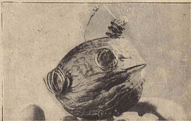
Kompletna stacja radjoodbiorcza w łupinie orzecha — została zmontowana przez amatorów w Berlinie.
