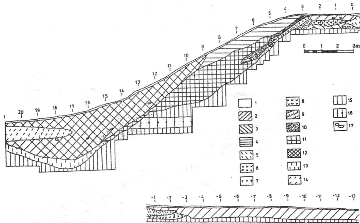
Fig. 29 - S III, profil estic: 1 - humus vegetal; 2 - ultimul nivel dacic; 3 - prima fază a locuinței de pe val; 4 - pământ brun din mantaua valului; 5 - lut galben-marونیu din panta interioară a valului; 6 - pământ negricios cu pietriș și piatră sfărâmată; 7 - lut depus în locuință; 8 - lut galben deschis; 9 - lut brun-gălbui; 10 - lut cu pietriș și nisip; 11 - pământ cu mult pietriș; 12 - pământ negru (din umplutura șanțului); 13 - pământ brun-negricios; 14 - pământ galben nisipos; 15 - lut galben (steril); 16 - pietriș (steril); 17 - pietre.
