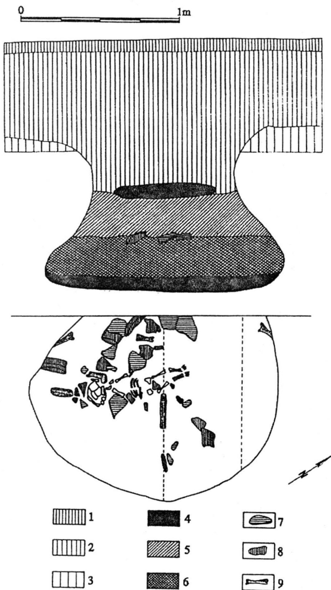
Fig. 93 - G11/92, plan și profil: 1 - humus vegetal; 2 - nivel dacic; 3 - lut galben (steril); 4 - cenușă; 5 - "capac" de lut; 6 - pământ de umplură; 7 - pietre; 8 - ceramică; 9 - oase de animale.
