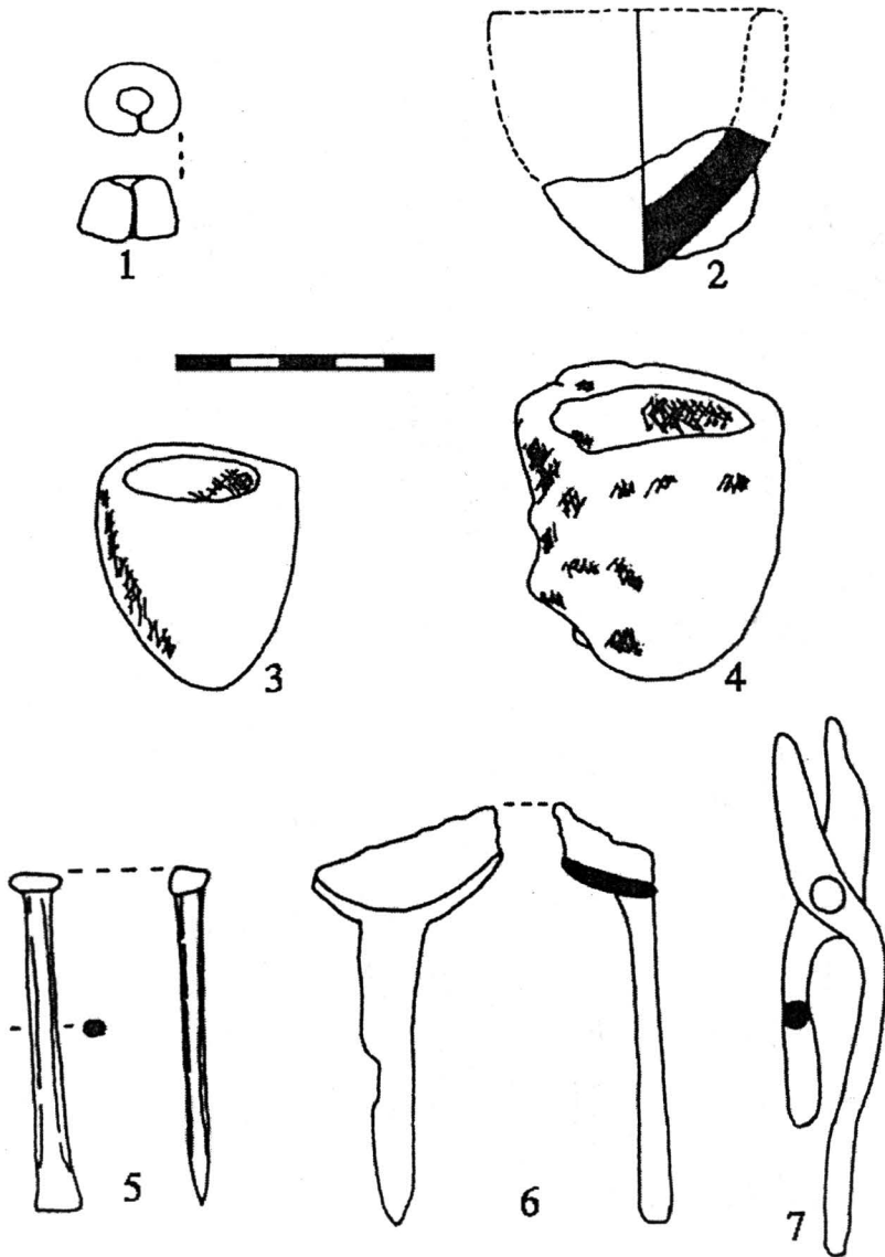
Fig. 113 - Creuzete ceramice (2-4) și unelte metalurgice din fier (1, 6-7) și bronz (5): 1, 6 din G5/95, 2 din L1/94, 3-5, 7 din săpăturile lui C.Seraphin (3-4 după fișele de inventar ale Muz. Sighișoara).
