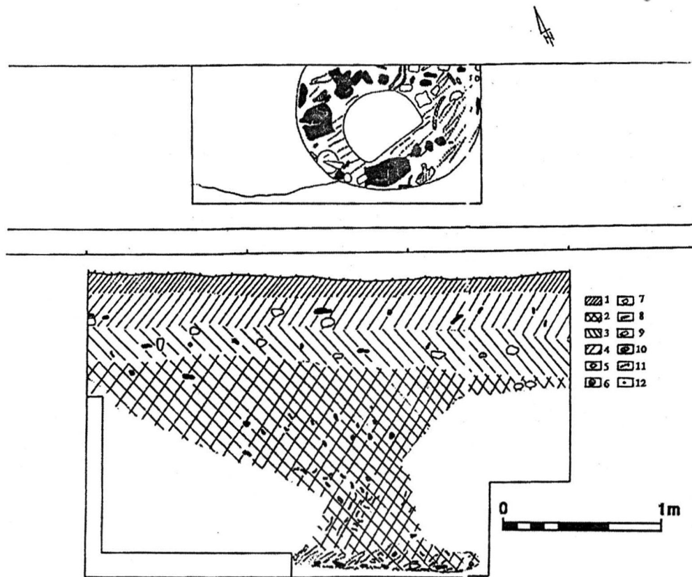
Fig. 97 - G15/91, plan și profil: 1 - humus vegetal; 2 - umplutura gropii 15/91; 3 - L3/91 (prima fază); 4 - L3/91 (a doua fază); 5 - pietre; 6 - ceramică; 7 - lespede de piatră de pe fundul gropii; 8 - oase de animale; 9 - lipitură de lut; 10 - bucăți de vatră; 11 - cenușă; 12 - verigi de coasă din fier.
