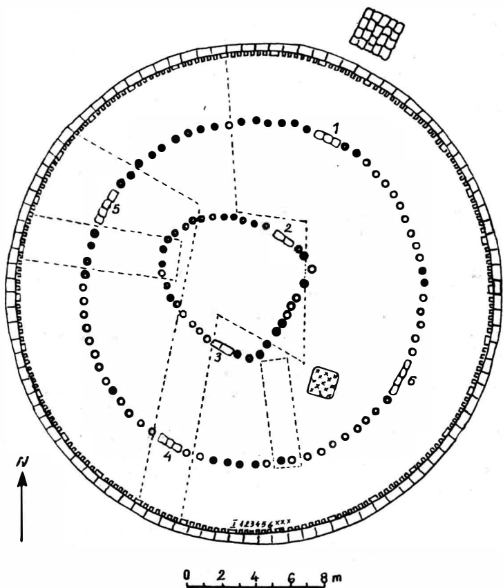
Fig. 54 : Planul marelui sanctuar circular (sanctuarul-calendar) de la Sarmizegetusa
