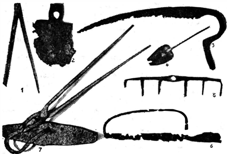
Fig. 40 : Unelte dacice de fier : 1. Compas ; 2. Sapă ; 3. Coasă ; 4. Lingură de fierar ; 5. Greblă ; 6. Ferăstrău ; 7. Clești și nicovală
