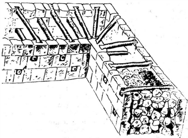
Fig. 22 : Structura zidului dacic (reconstituire)
