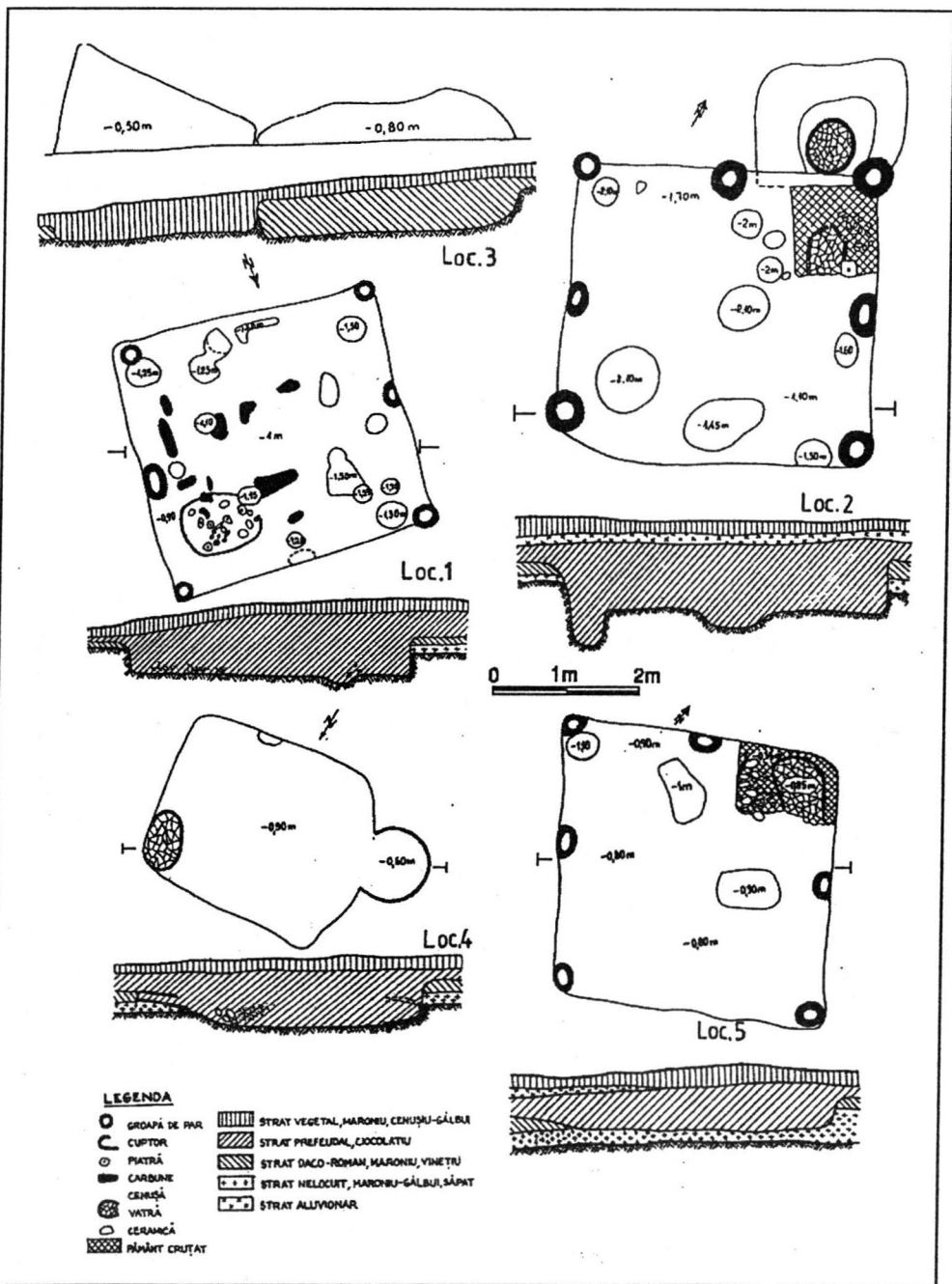
4. Gura Gurgotei. Planurile locuințelor nr. 1-5.
