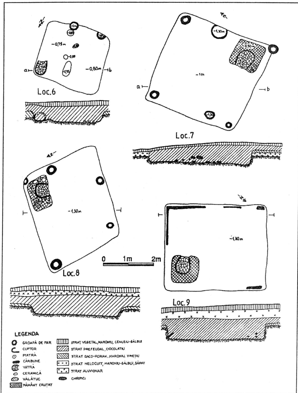
5. Gura Gurgotei. Planurile locuințelor nr. 6-9.
