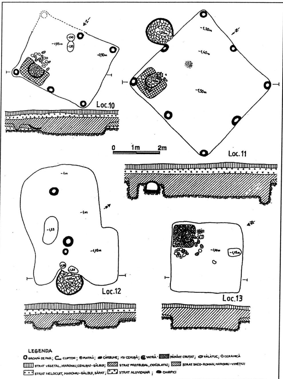
6. Gura Gurgotei. Planurile locuințelor nr. 10-13.
