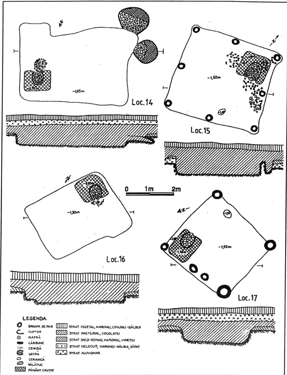
7. Gura Gurgotei. Planurile locuințelor nr. 14-17.
