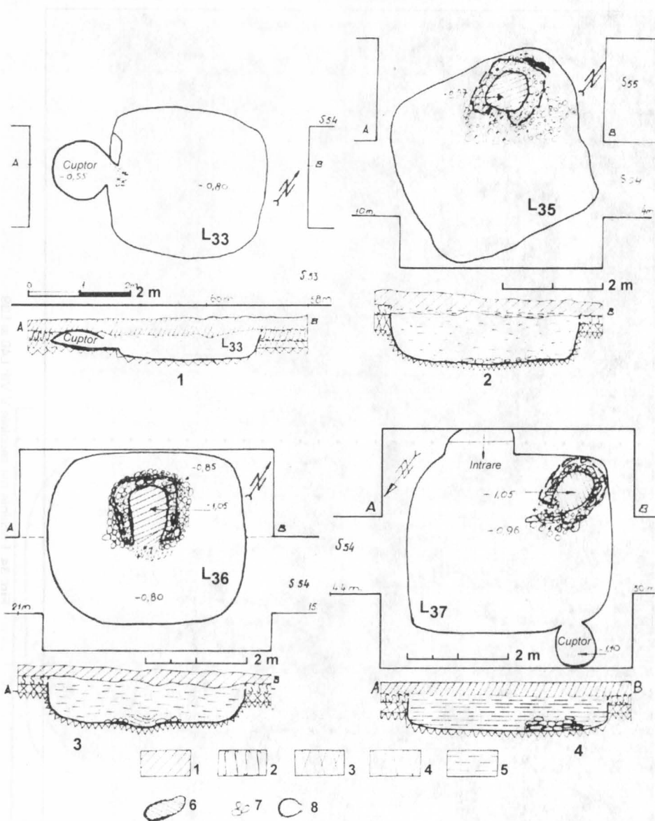
Fig. 33. Planuri și profile de locuințe din secolele V-VIII: 1 - L33; 2 - L35; 3 - L36; 4 - L37.
