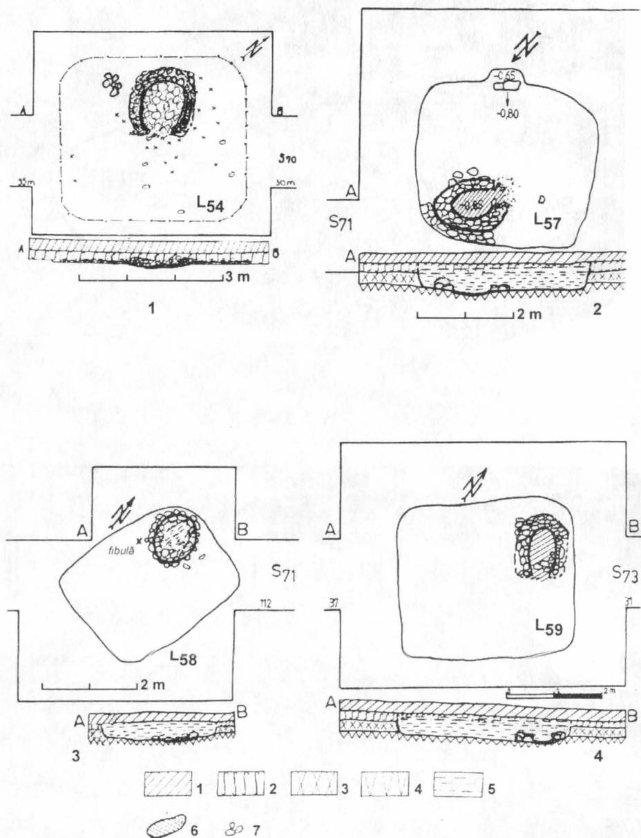
Fig. 44. Planuri și profile de locuințe din secolele V-VII: 1 - L54; 2 - L57; 3 - L58; 4 - L59.
