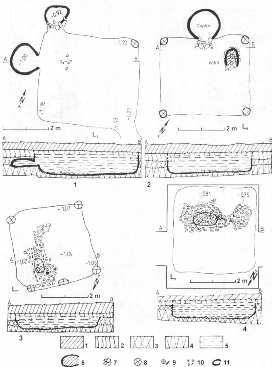
Fig. 23. Planuri și profile de locuințe din secolele V-VII: 1 - L5; 2 - L6; 3 - L7; 4 - L8.
