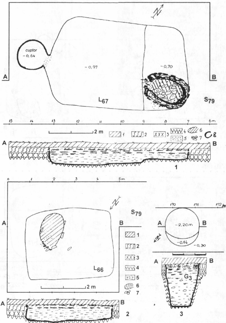
Fig. 49. Planuri și profile de locuințe și gropi de provizie (3), din secolele V-VII: 1 - L67; 2 - L66; 3 - G3. Legenda: 1 - sol vegetal; 2 - strat brun mazăros (nivel sec. V-VIII); 3 - strat cafeniu (nivel preistoric); 4 - pământ galben; 5 - umplutura locuințelor; 6 - vatră simplă sau vatră de cuptor din piatră; 7 - pietre; 8 - cuptor din lut.
