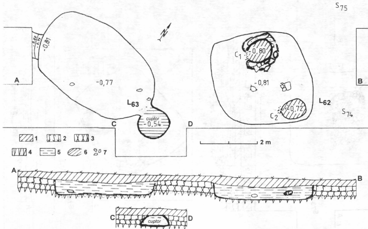
Fig. 46. Planuri și profile de locuințe din secolele V-VII (L63) și din sec. VII-VIII (L62).
