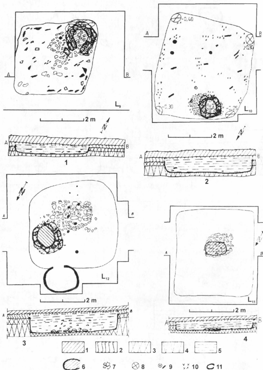
Fig. 24. Planuri și profile de locuințe din secolele V-VII: 1 - L9; 2 - L10; 3 - L12; 4 - L11.
