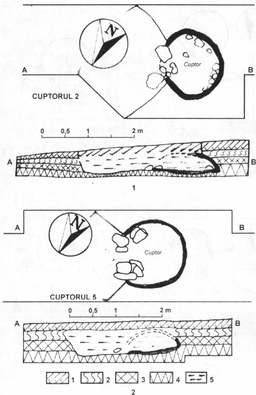
Fig. 58. Planuri și profile de cuptoare de copt, din secolele V-VII: 1 – C2, 2 – C5.
