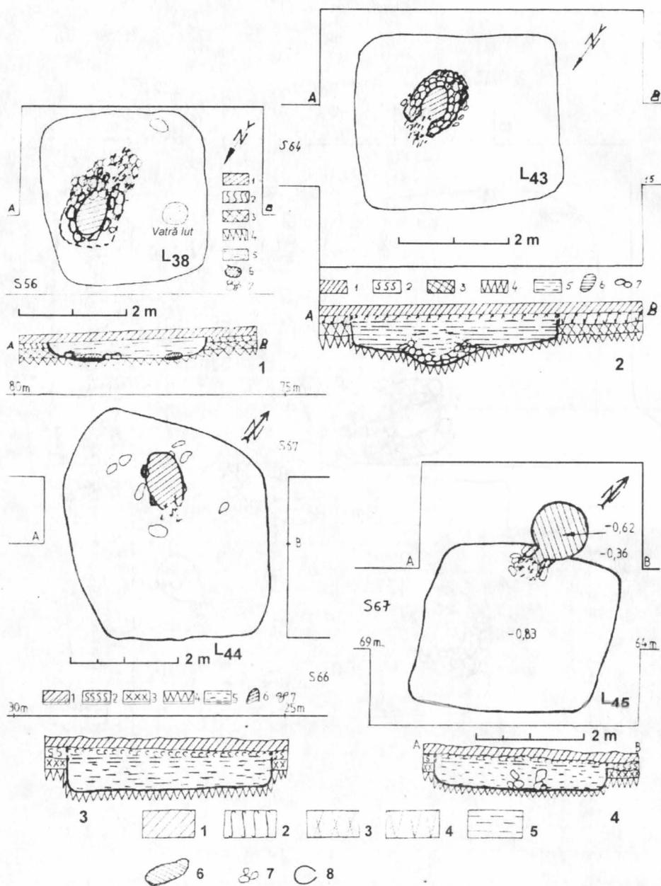
Fig. 38. Planuri și profile de locuințe din secolele V-VII: 1 - L38; 2 - L43; 3 - L44; 4 - L45.
