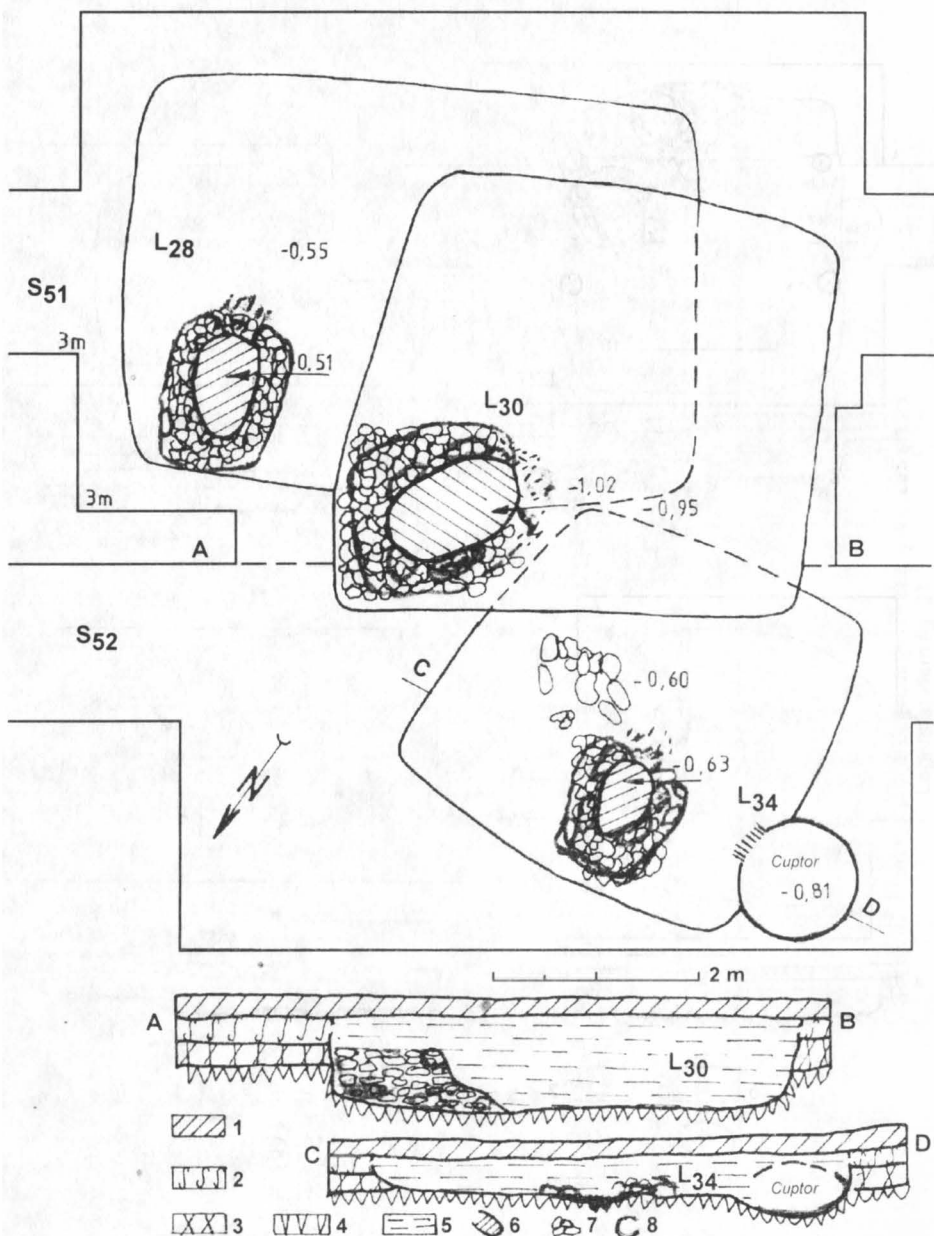
Fig. 32. Planuri și profile de locuințe din sec. V-VII: L28, L30 și L34.
