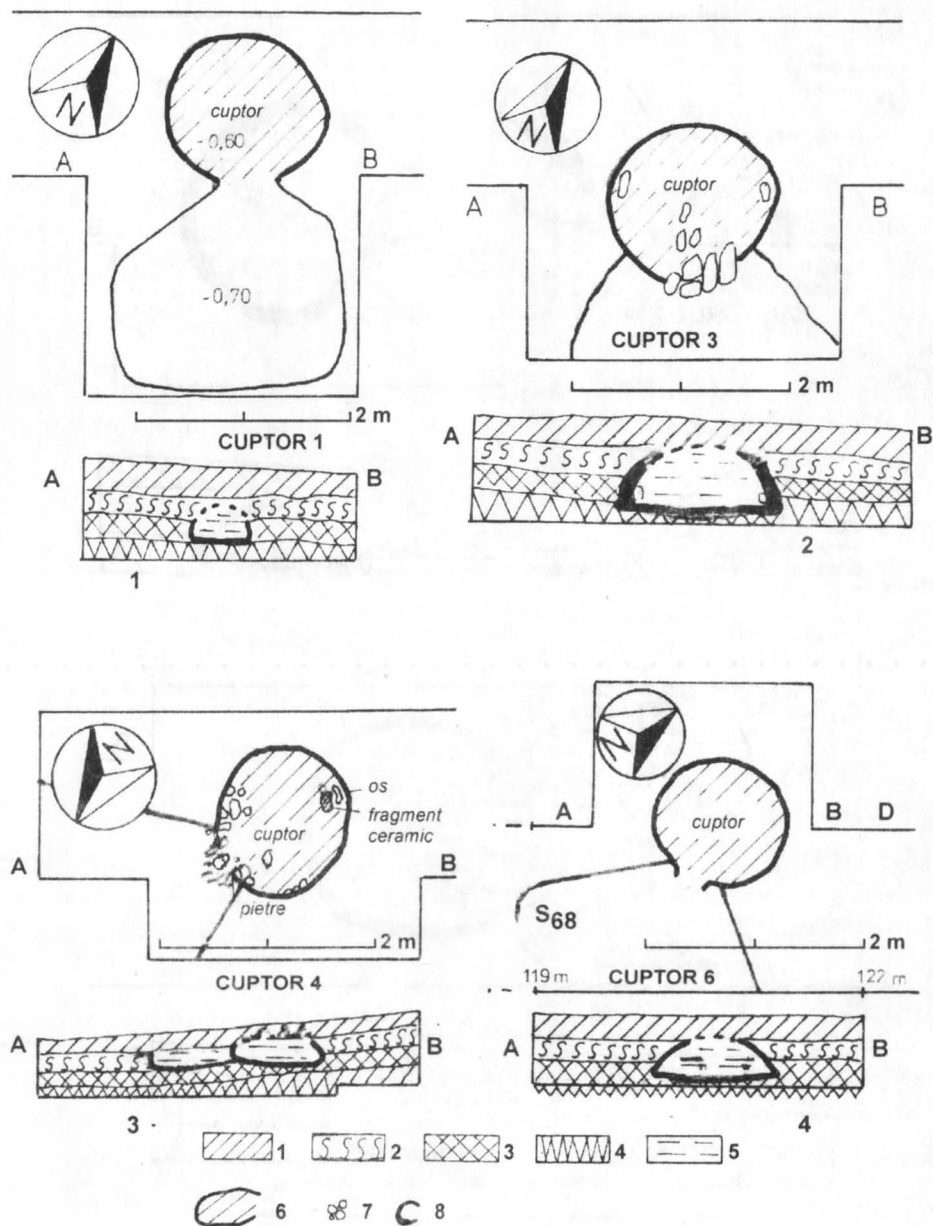
Fig. 57. Planuri și profile de cuptoare de copt pâine, din secolele V-VII: 1 - C1, 2 - C3; 3 - C4; 4 - C6. Legenda: 1 - sol vegetal; 2 - strat brun măzăros (nivel sec. V-VIII); 3 - strat cafeniu (nivel preistoric); 4 - pământ galben; 5 - umplutura locuințelor; 6 - vatră simplă sau vatră de cuptor din piatră; 7 - pietre; 8 - cuptor din lut.
