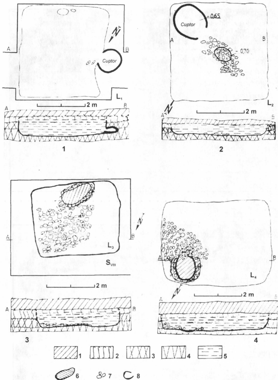
Fig. 21. Planuri și profile de locuințe din secolele V-VII: 1 - L1; 2 - L2; 3 - L3; 4 - L4.
