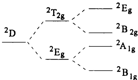
Fig. 28. Scindarea termenilor configurației d^9 în câmp tetragonal
