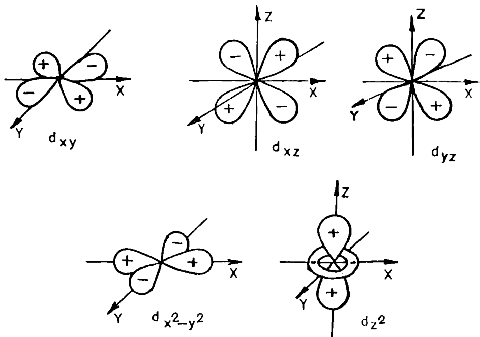
Fig. 3. Représentarea spațială a orbitalelor d
