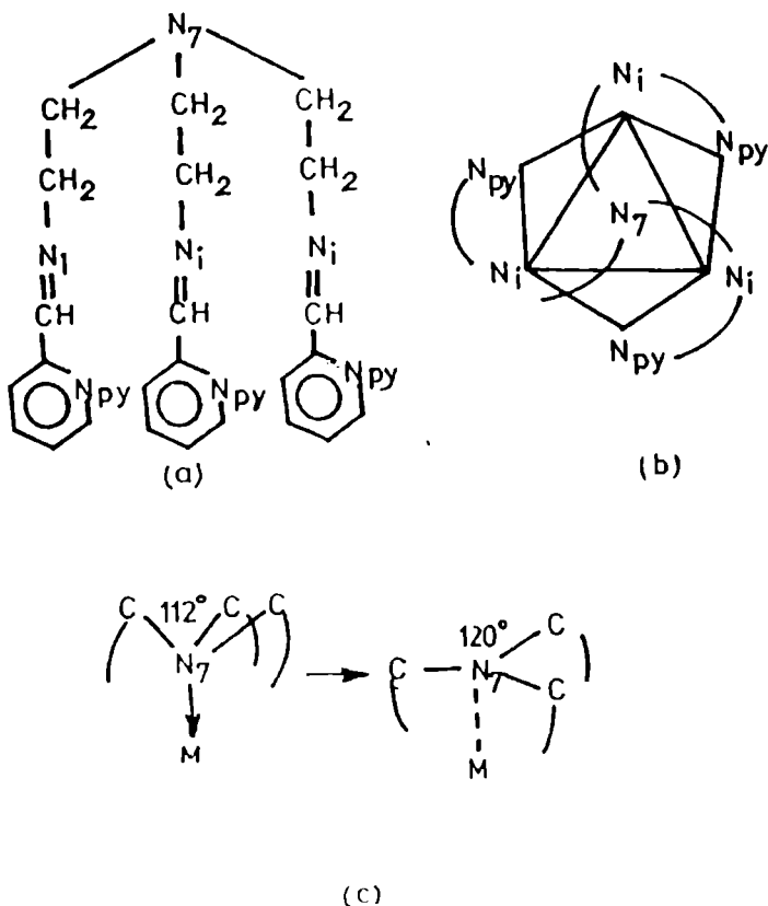
Fig. 34. a) Ligandul „trenpy”; atomii de azot sunt notați N_{py} (azot piridinic), N_i (azot iminic), N_7 (al șaptelea atom de azot); b) reprezentarea combinației complexe [M(\text{trenpy})]^{2+} c) modificarea unghiului C - N_7 - C când nivelele t_{2g} sunt ocupate cu electroni
