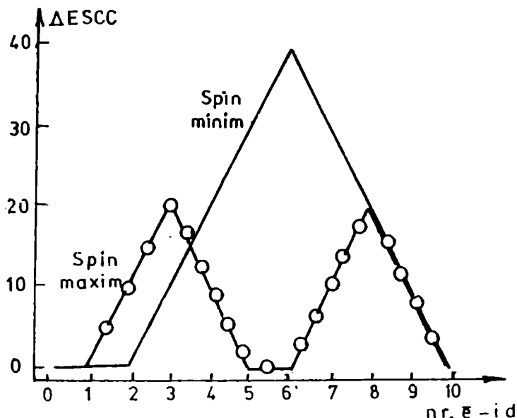
Fig. 32. Stabilitatea relativă a coordinerii octaedrice față de cea trigonal-prismatică în funcție de configurația d^n
