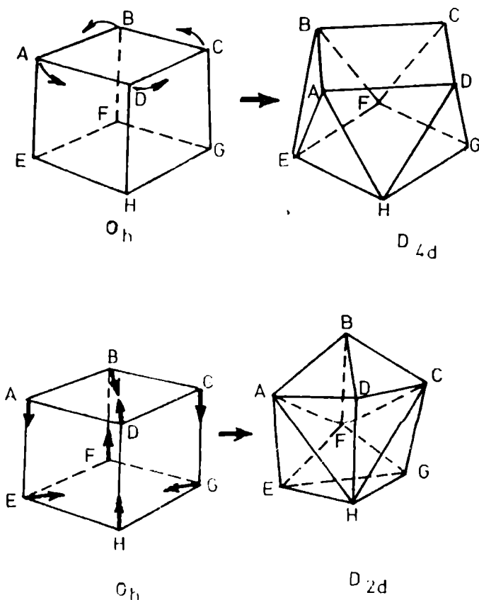
Fig. 35. Poliedrele de coordonare pentru numărul de coordonare 8
