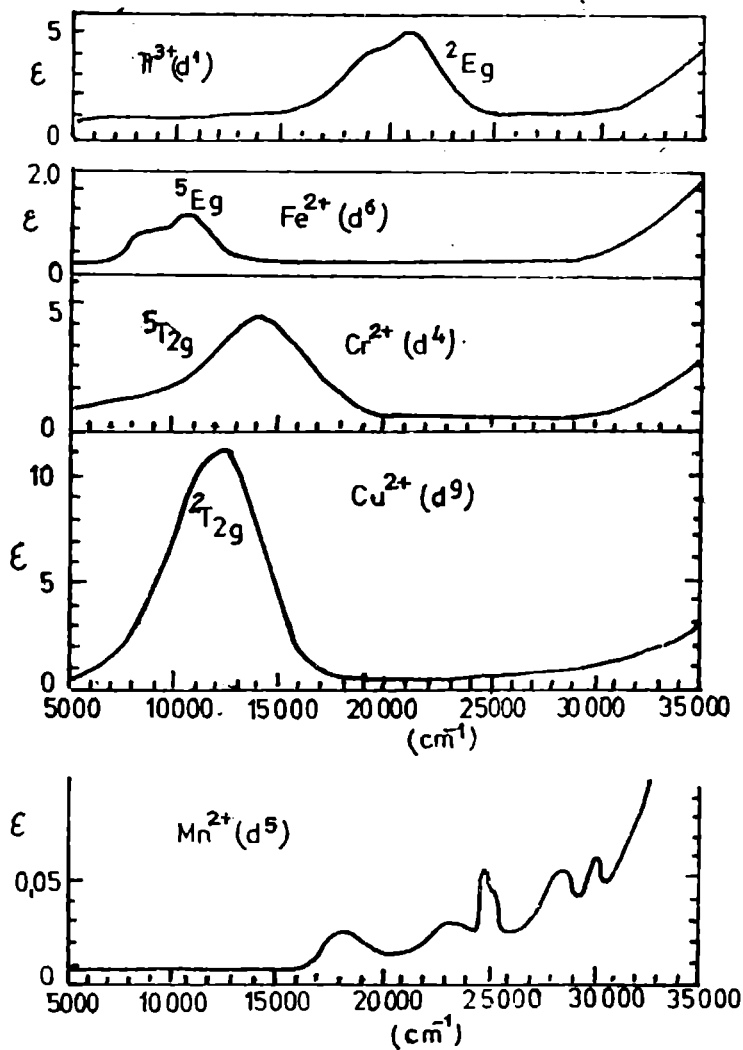
Fig. 24. Spectrele electronice ale ionilor [M(H_2O)_6]^{2+} în domeniul 5000 - 35000\text{ cm}^{-1}
