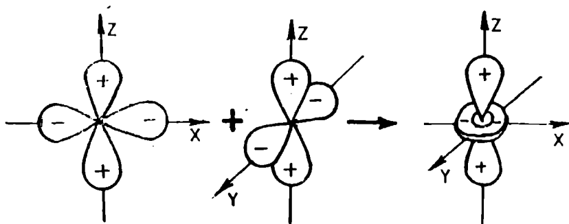
Fig. 4. Reprezentarea orbitalei d_{xy} ca o combinație lineară a orbitalelor d_{z^2-x^2} și d_{z^2-y^2}
