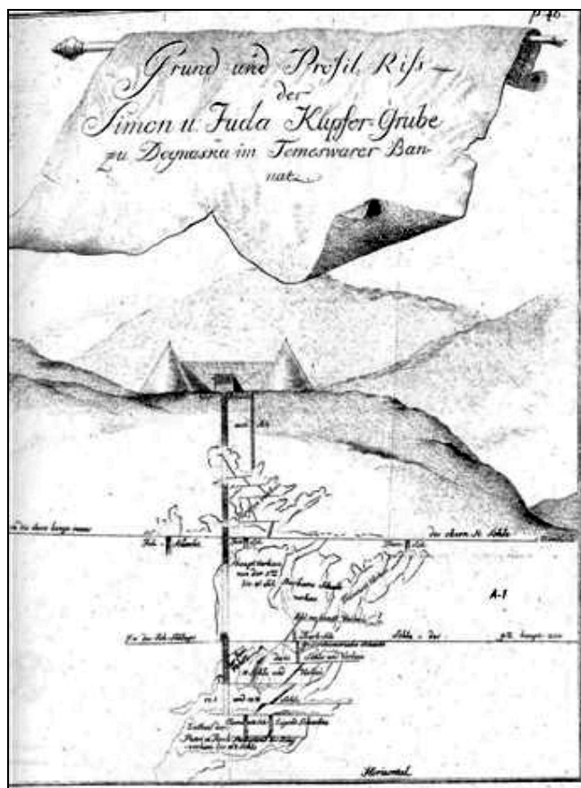
Fig. 10. Schița minelor Simon și Judea din Dognecea
