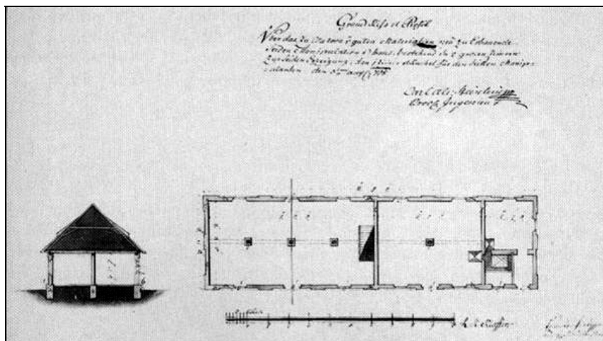
Fig. 86. Planul Manufacturii pentru prelucrarea gogoșilor de mătase din Ciacova. 1768
