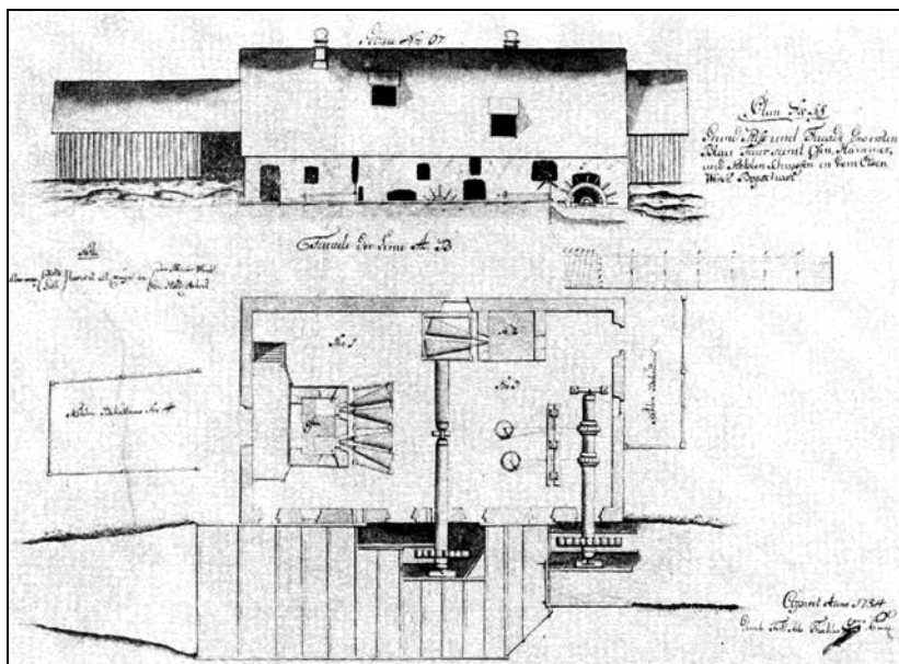
Fig. 12. Atelierul din Bocșa. 1784
