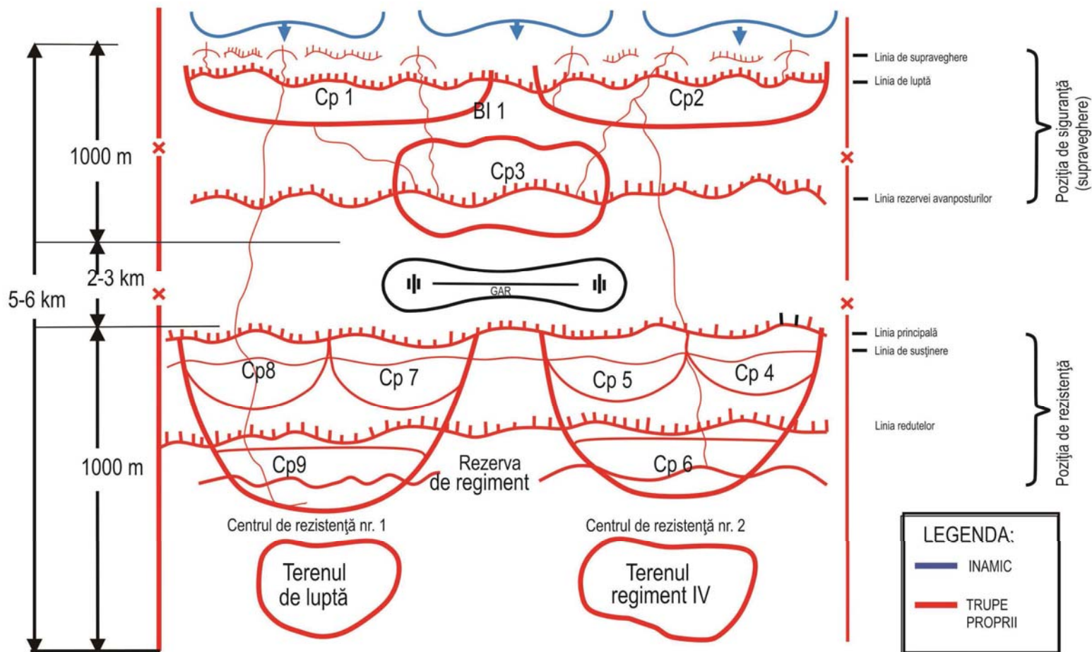
Schema nr. 6: DISPOZITIVUL REGIMENTULUI DE INFANTERIE ÎN APĂRARE (PERIOADA INTERBELICĂ)
