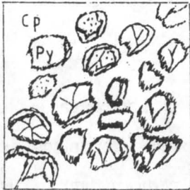
Pirită casantă în calcopirita plastică
