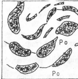
Incluziuni de silicați în pirotină deformată
