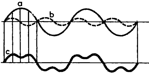
Р и с. 3 Схема сложного звука: a – основной тон, b – обертон, c – сложный звук.
