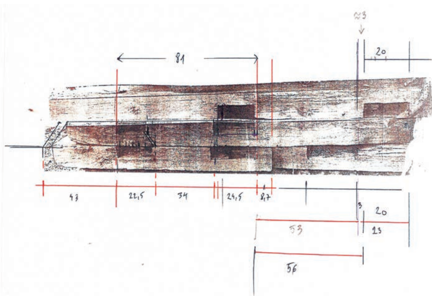
Fig. G. Pe linia roșie, dimensiunile reale ale grinzii-mamă.
