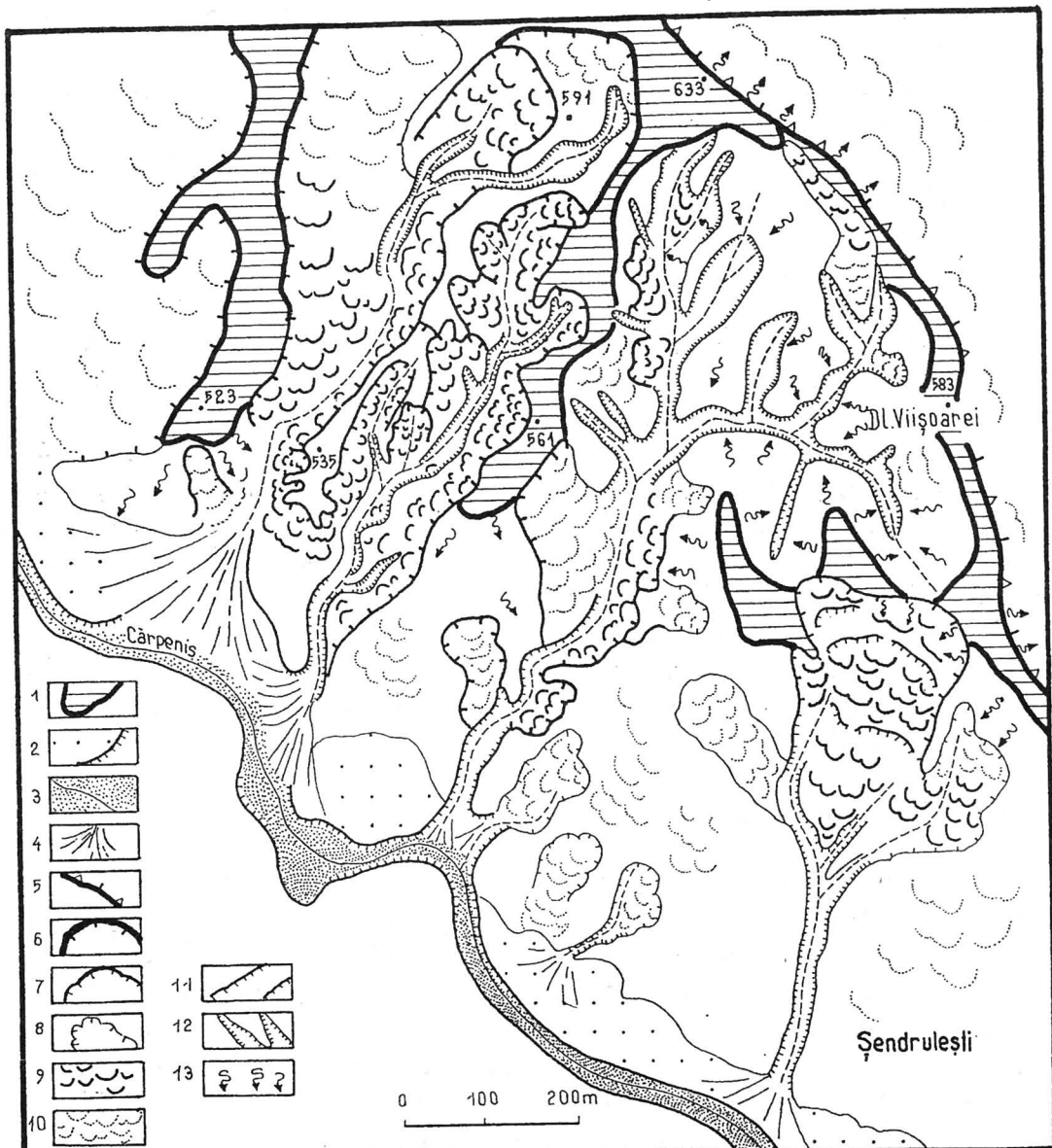
1. suprafețe interfluviale, 2. lunca, 3. albia minoră, 4. con de dejecție, 5. frunte de cuestă 6. ripă de desprindere principală, 7. ripă de desprindere secundară activă, 8. alunecare de vale 9. vâluri recente de alunecare, 10. vâluri vechi, fixate, de alunecare, 11. trepte de alunecare 12. ravene și ogăse cu maluri abrupte, 13. sîroiri.
