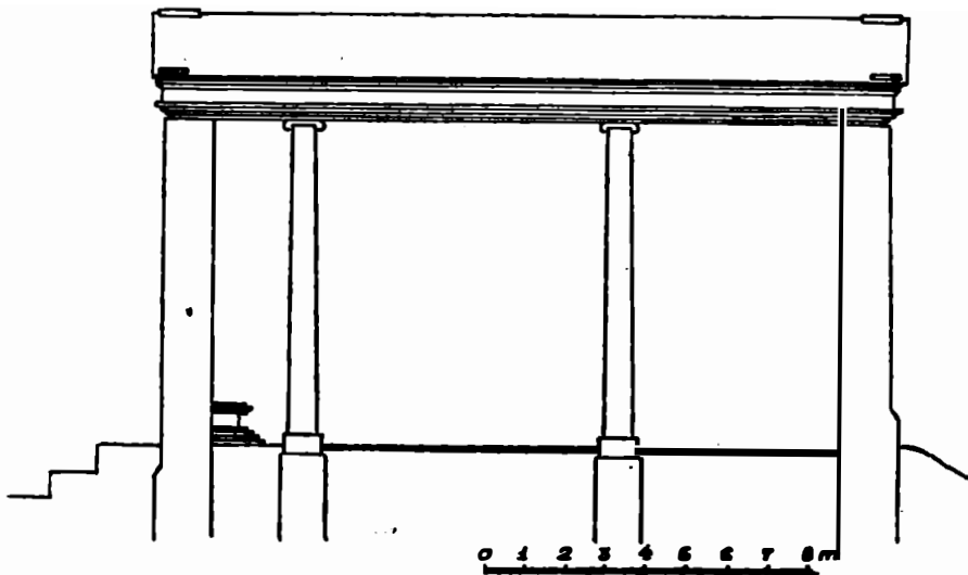
Sectiune longitudinală prin templul zeilor sirieni de la Sarmizegetusa (Reconstituire)
