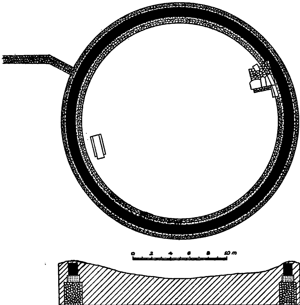
Planul Mausoleului Aureliilor de la Sarmizegetusa
