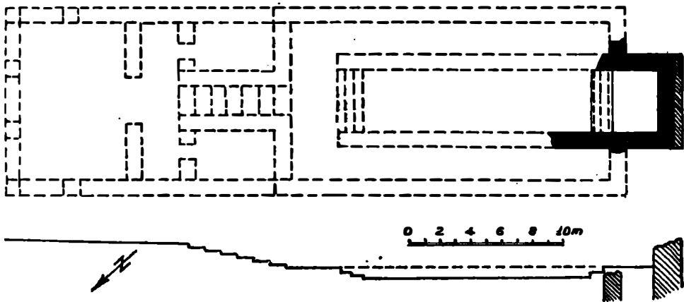
Planul (reconstituit) al mithraeum-ului de la Sarmizegetusa
