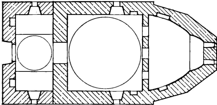
Fig. 5. -- Mănăstirea Frăsinei. Planul bisericii vechi.
