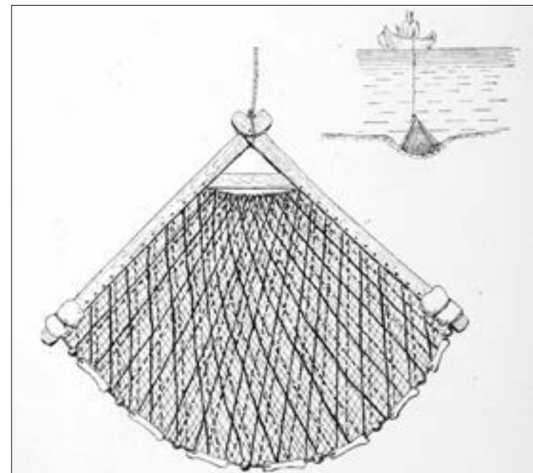
Trandadaia și modul cum se pescuiește cu ea în fundul Dunării.
