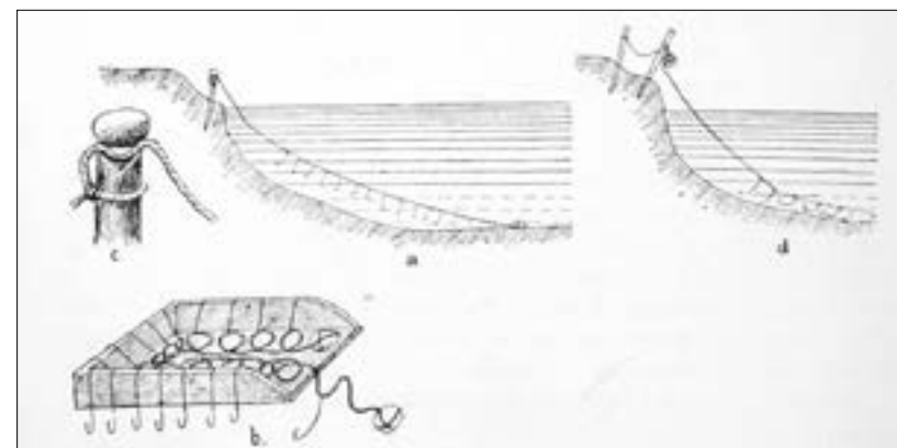
Priponul simplu; a) Modul cum se așază priponul în apă; b) Masa cârligelor; c) Parul crestat în cap, cu streaja; d) Pripon cu clopoțel.
