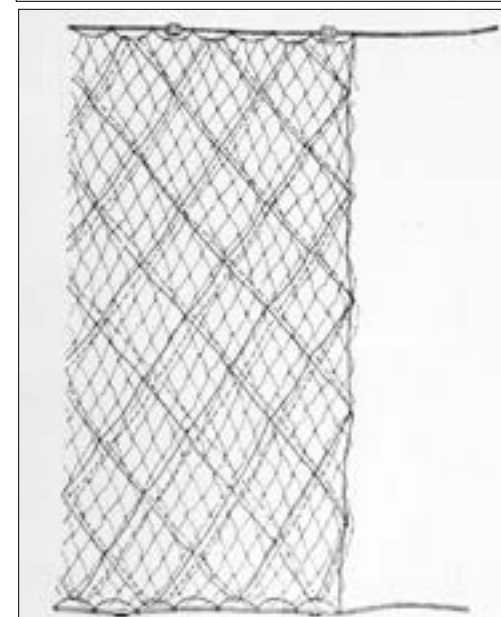
Trandadaia și modul cum se pescuiește cu ea în fundul Dunării.
