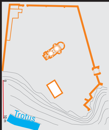
📍 Biserica „Buna Vestire” („Răducanu”). Plan de situație
