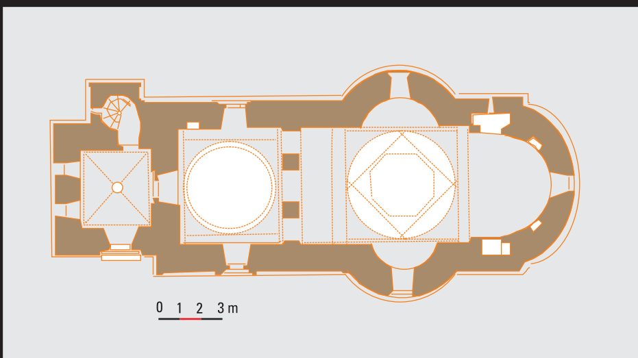
📍 Biserica „Buna Vestire” („Răducanu”). Plan
