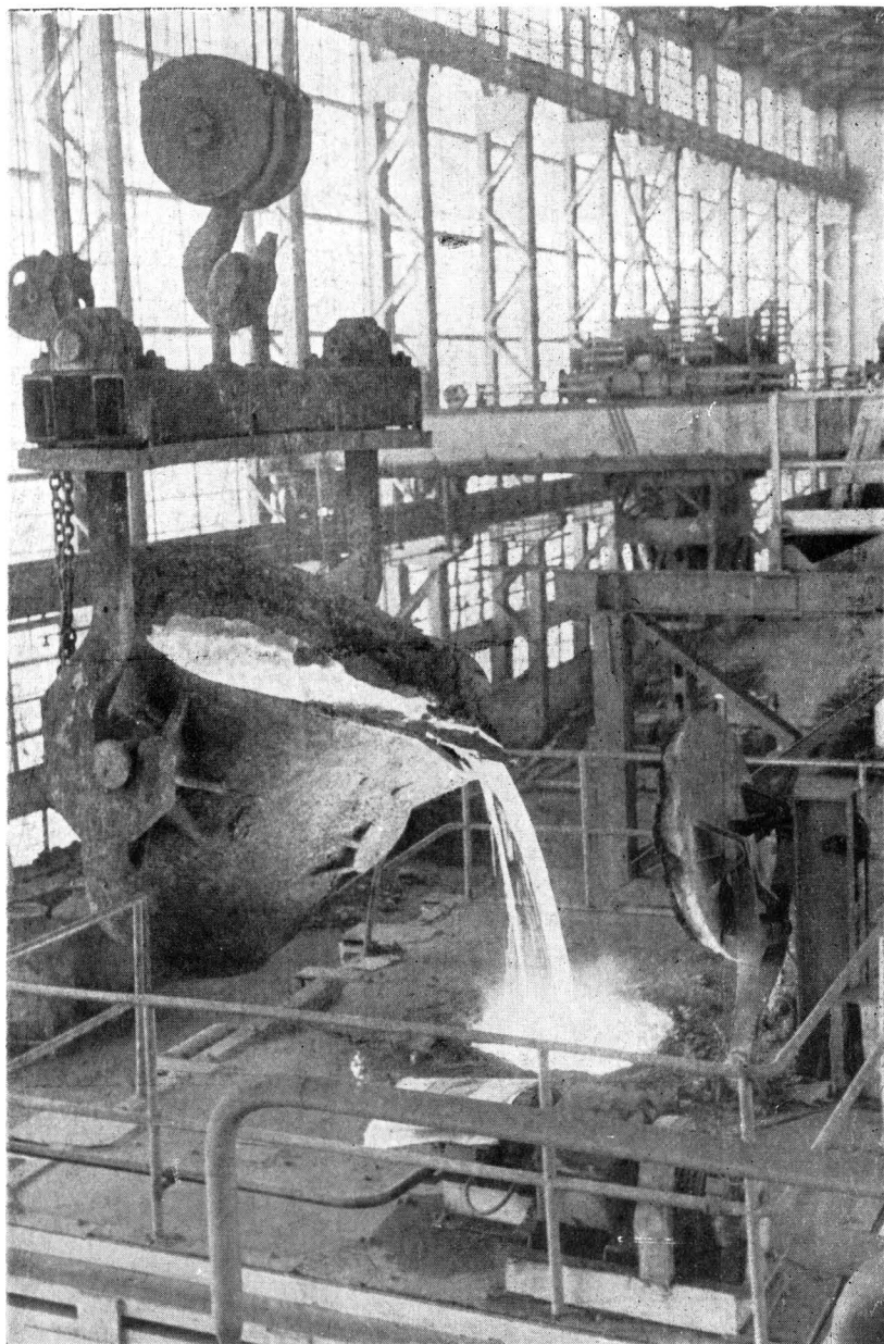
26. Turnarea cuprului la Combinatul chimico-metalurgic din Baia Mare.
