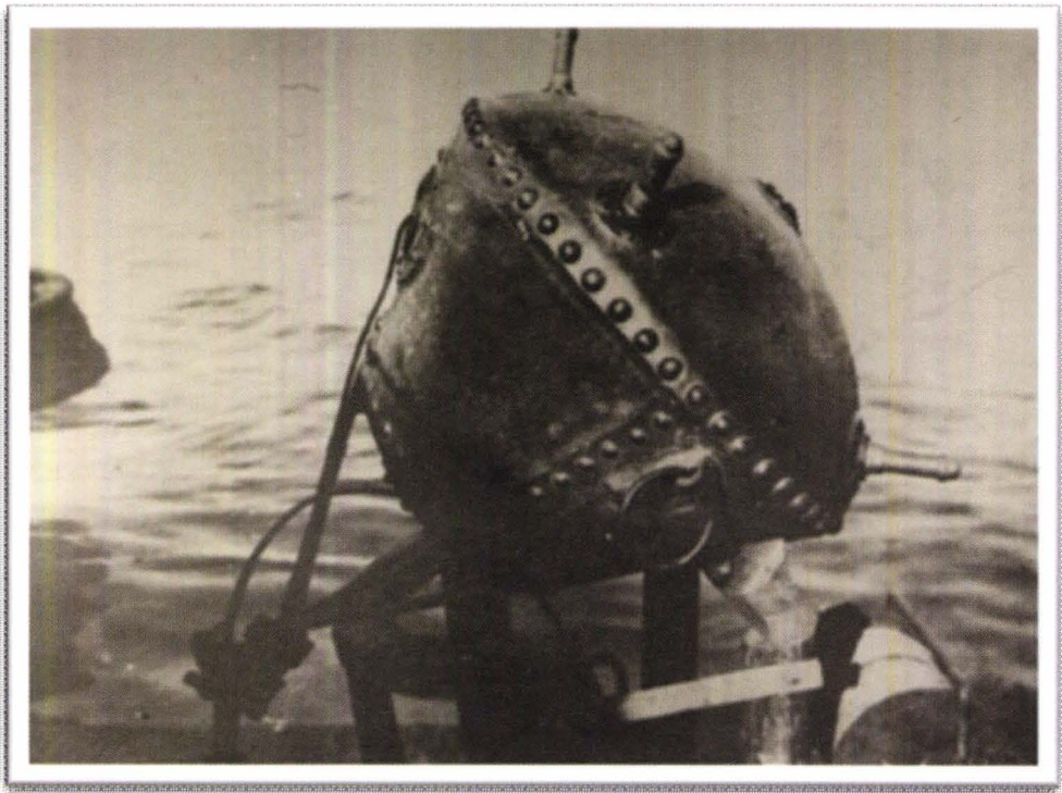
Mină sistem „Hertz”, din dotarea Marinei Militare Române, care s-a folosit și în timpul Primului Război Mondial
