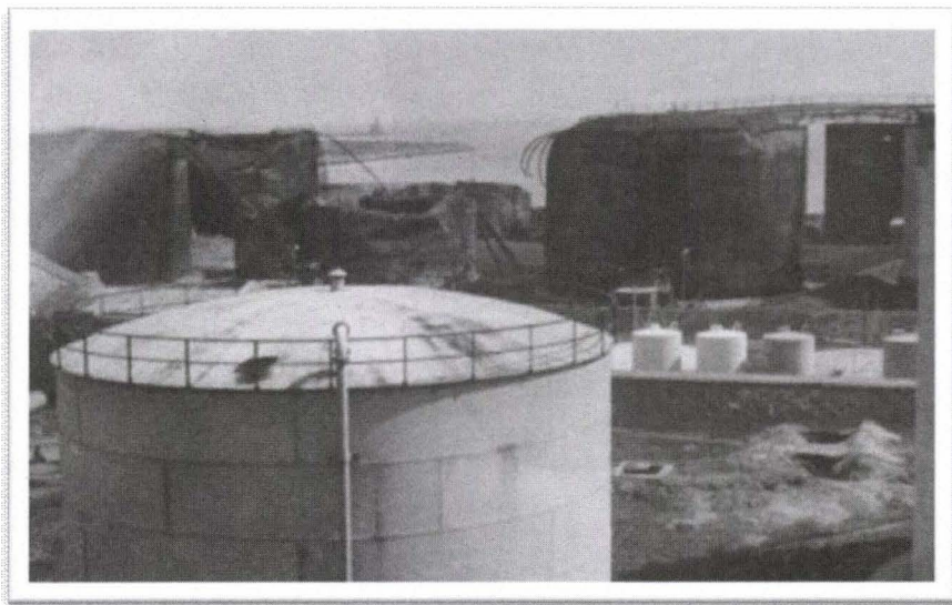
Constanza, Petroleumtank im Hafen
