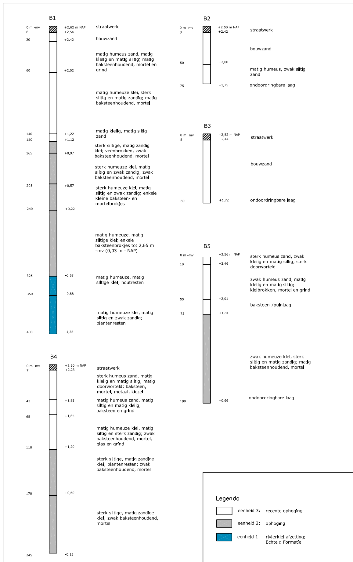
Afb. 3: Boorstaten, boringen 1 t/m 5.
