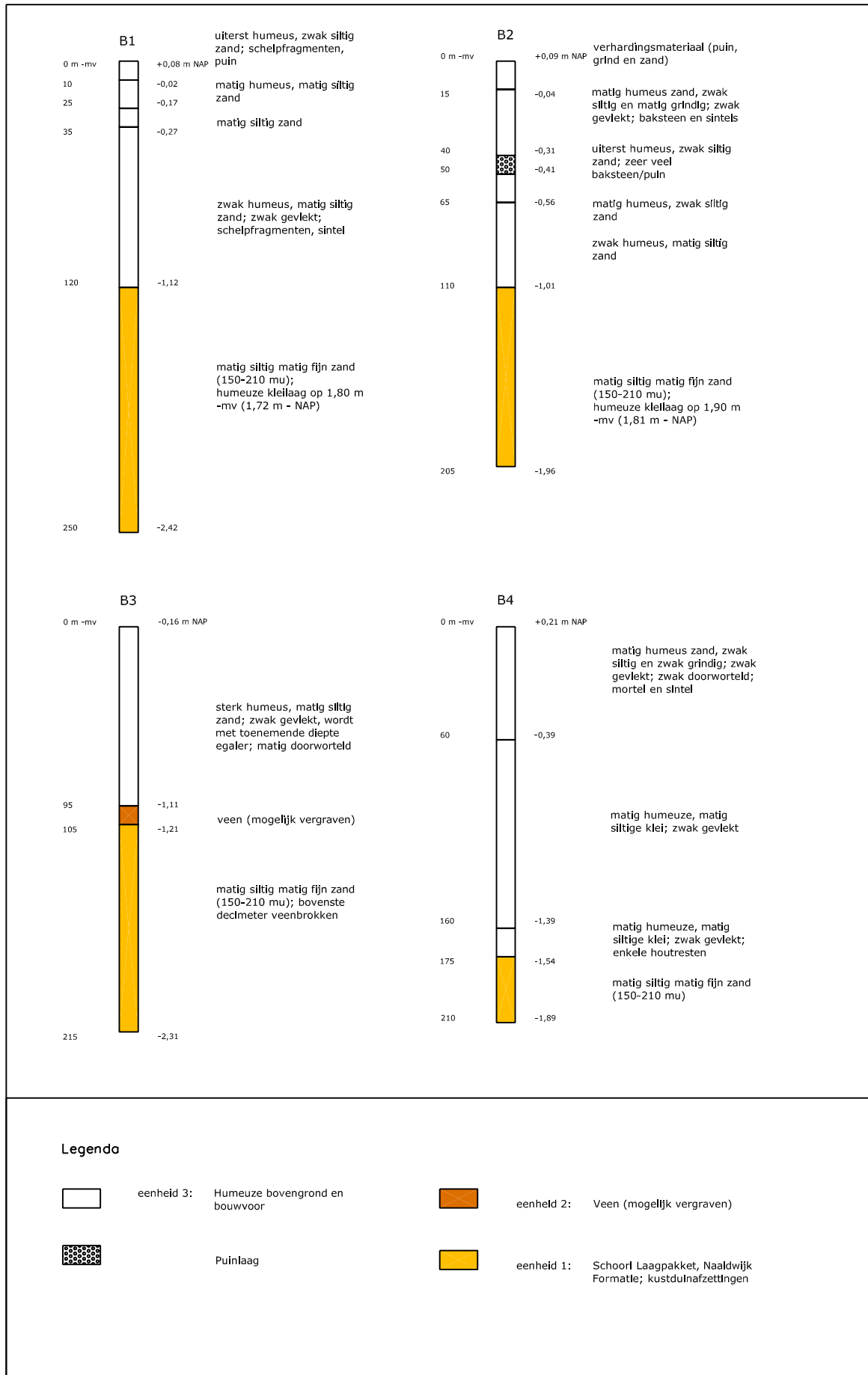
Afb. 3: Boorstaten, boringen 1 t/m 4.
