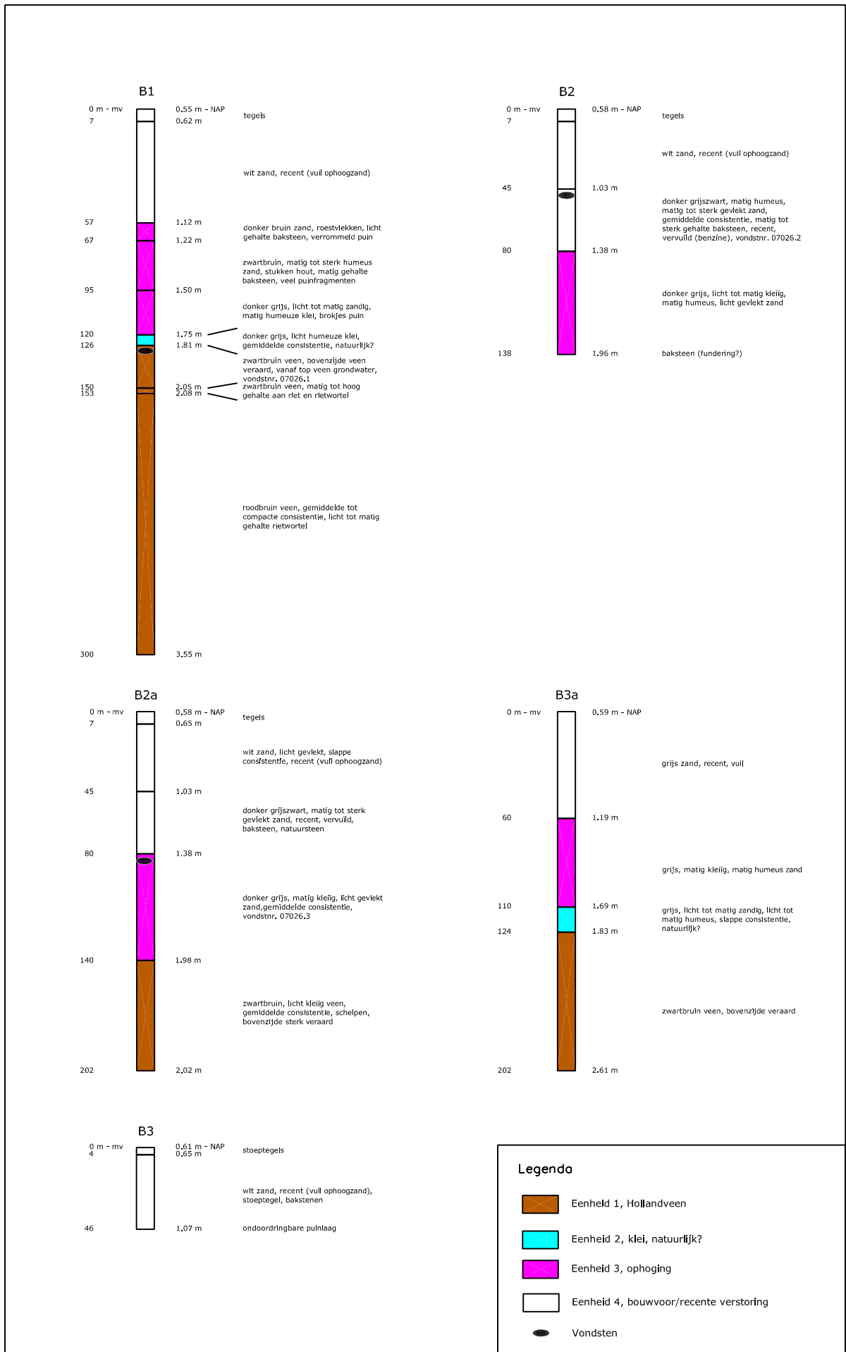
Afb. 5: Boorstaten, boringen 1 t/m 3.
