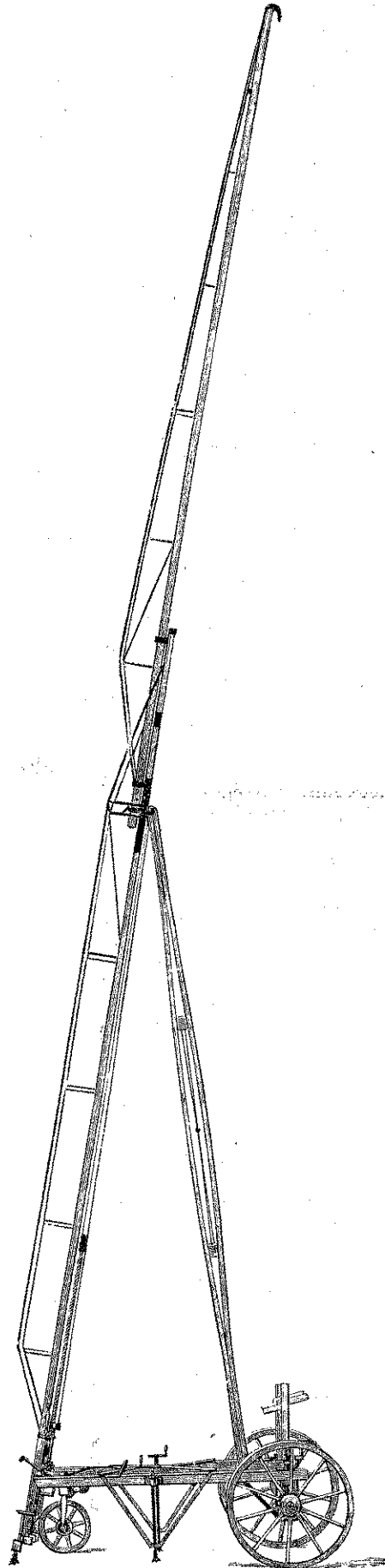
1. sz. ábra »E« létra teljes felállításban.
