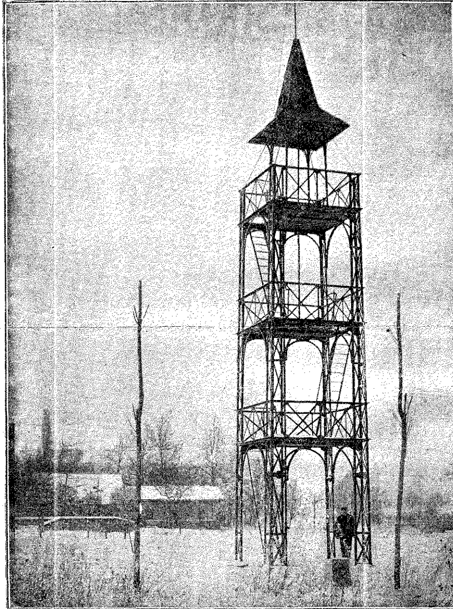
3 ábra. Az a'csuthi vas-mászótorony.
