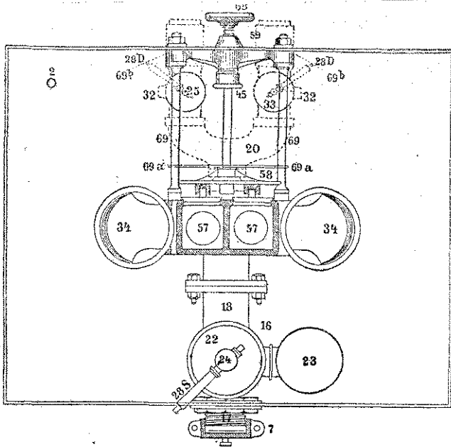
3 ábra. (Felülnézet).
