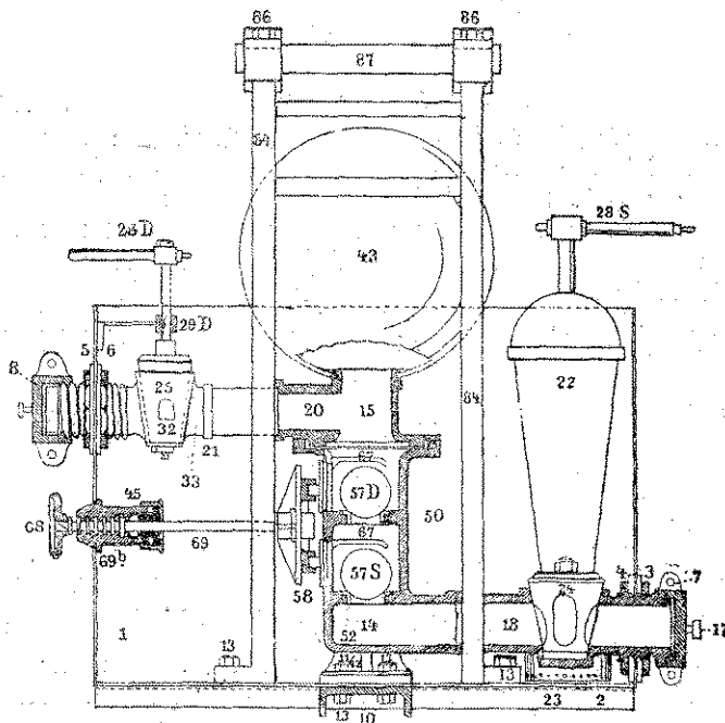
2. ábra. (Kereszmetszet.)
