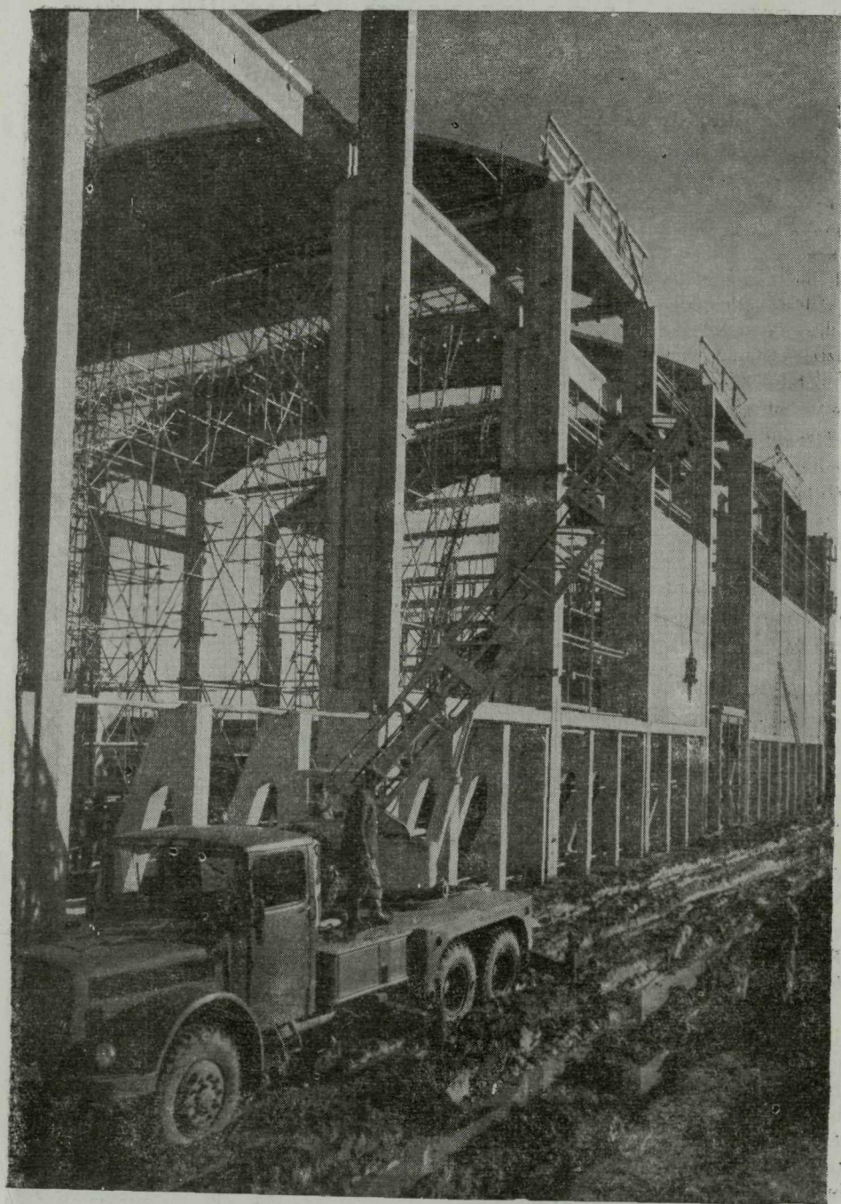
A szolnoki Tiszamenti Vegyiművek építése
