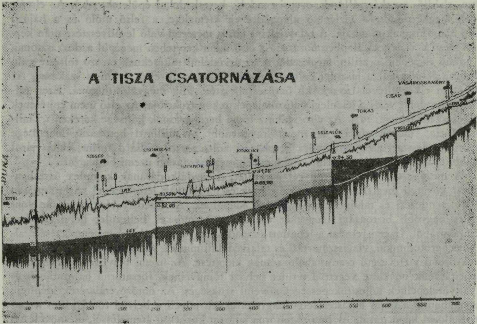
A Tisza csatornázása
