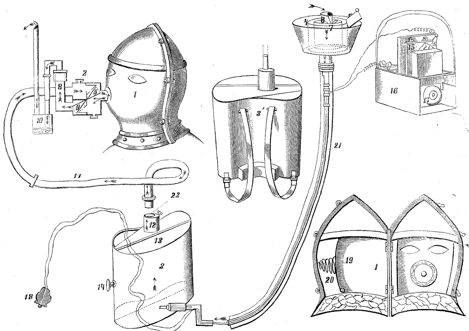
(Lélegzési készülék fojtó füstben és gásban.)
