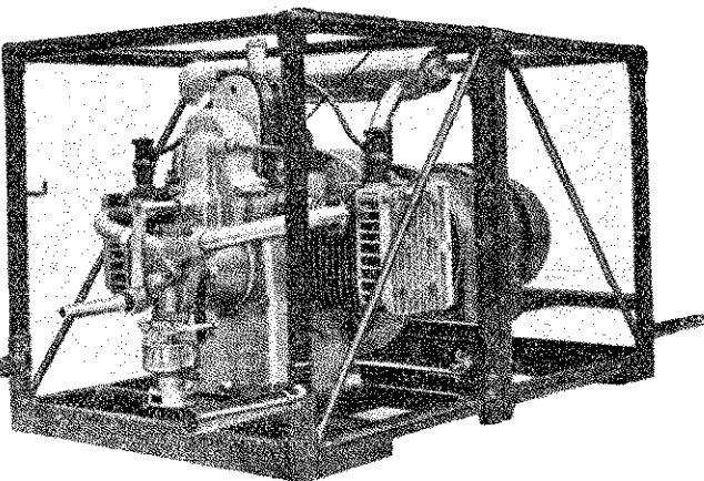
2. ábra. Csonka-féle motoros — hordozható, szétszerelhető — generátor.
