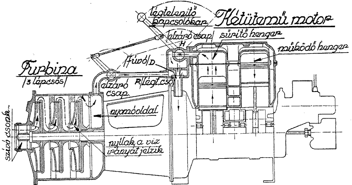
3. ábra. Szemléltető rajz az elvi elrendezés megértésére.
