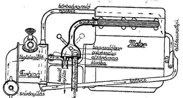
5. ábra. Négyütemű (szelepes) motor, kipuffogó gázokkal működtetett gázugár légszivattyús motorfecskendő szemléltető rajza.
