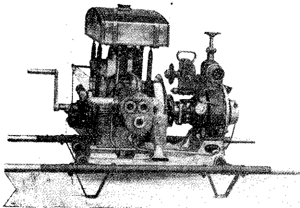
1. ábra. Csonka-féle magyar gyártmányú motorral felszerelt Mátrai-féle kismotorfecskendő.
