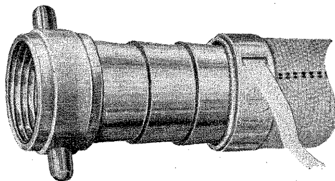
A szalaggal befűzött „KR”-gyűrűt felhúzzuk a tömlőre, azután a bekötendő csavar (apa- vagy anyarész), kapocs (storz) csonkját betoljuk a „KR”-gyűrűvel ellátott tömlőbe.
