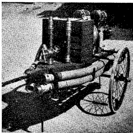
Tömlőtartóláda kismotorfecskendőre felszerelve
