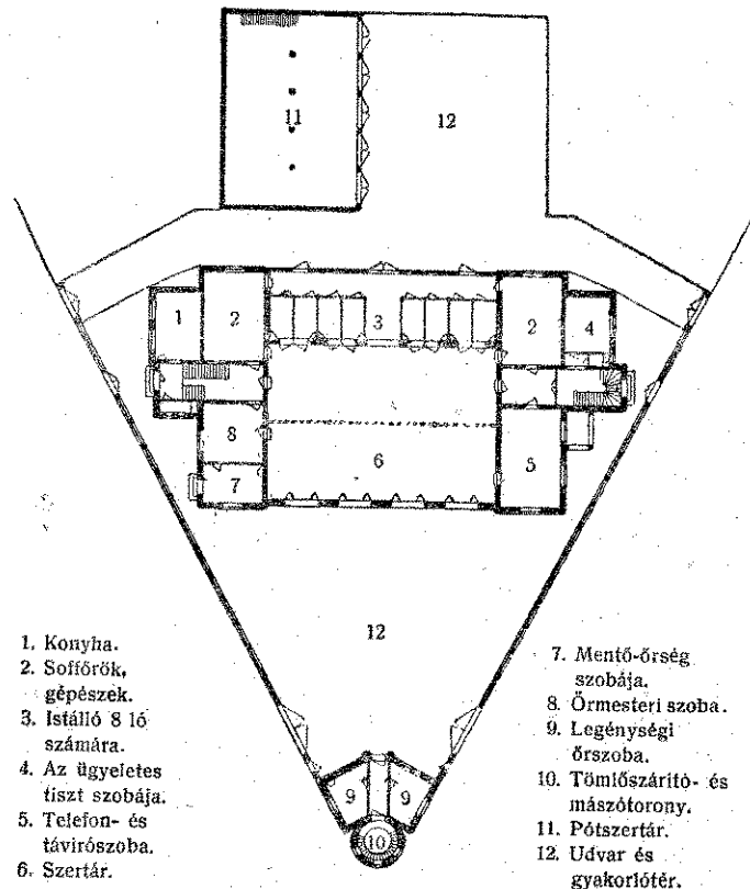
Bréma II. kerületi őrség épületének alaprajza.
