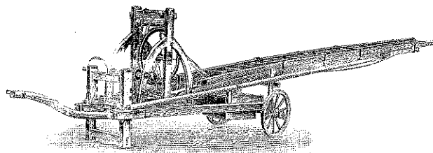
8. ábra. Ugyanez visszaszerelve.
