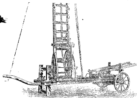
7. ábra. Ugyanez oldalállásban.
