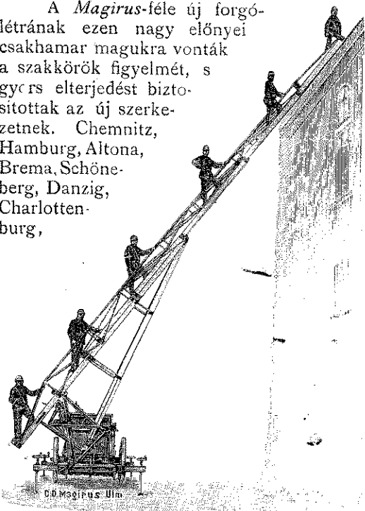
4. ábra. A létra oldalát hajlítva és házhoz támasztva.
