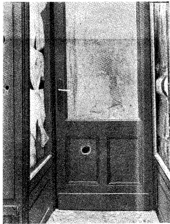
Az égő divatáru üzlet zárt bejárati ajtaja, a poroltókészülék sugáresővének bevezetésére készített kerek nyílással.
