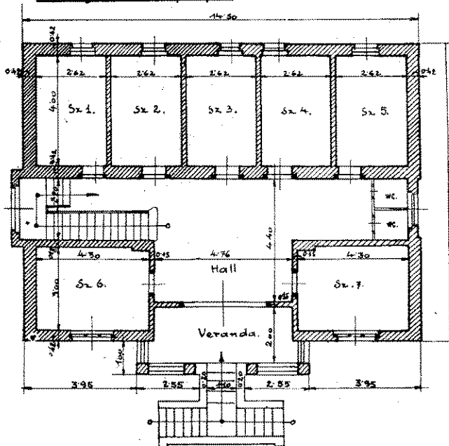
Földszíni alaprajz.
