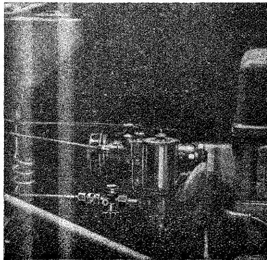
8. ábra. Hőhatásra záródó benzincsap autómotor karburátor előtt
