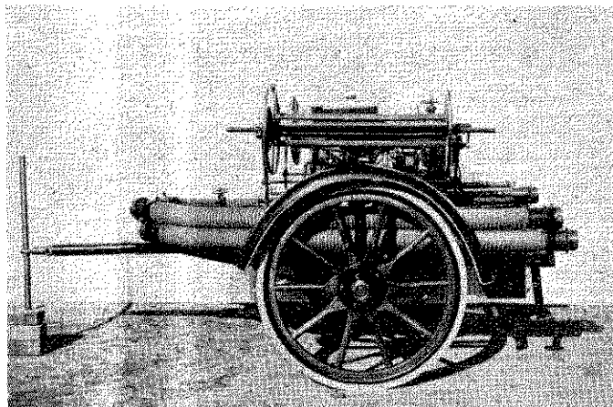
Mátrai kismotorfecskendő (négyütemű motor, tisztavíz hűtés, tengelykapcsoló, bronzszivattyú, 400 liter/8 atm. teljesítmény)
