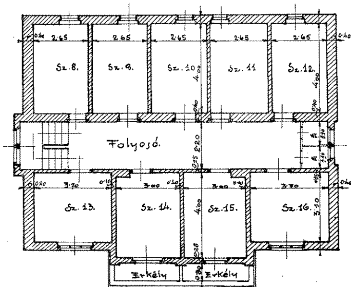
F.emeleti alaprajz.
