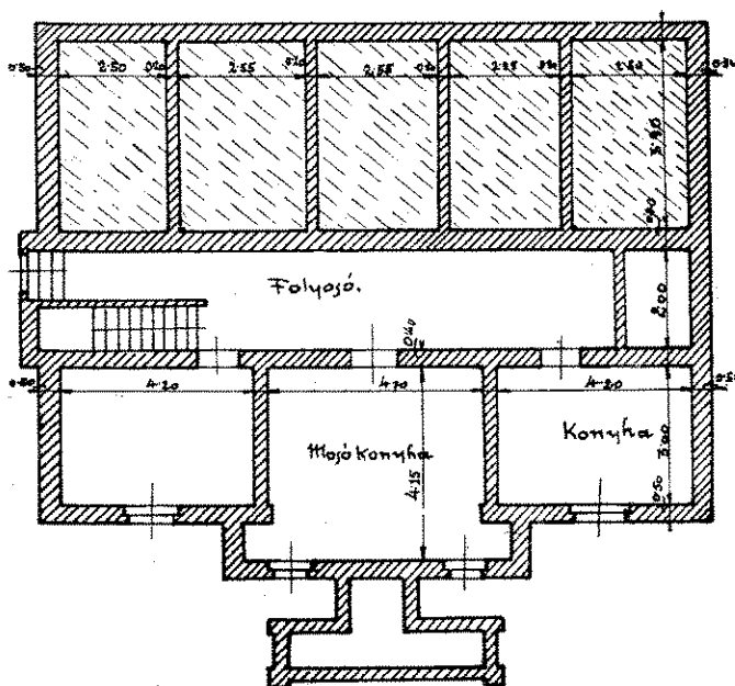
Pince alaprajz.
