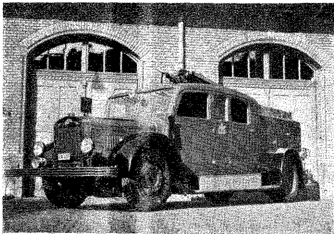
A „Turul“ autófecskenő
