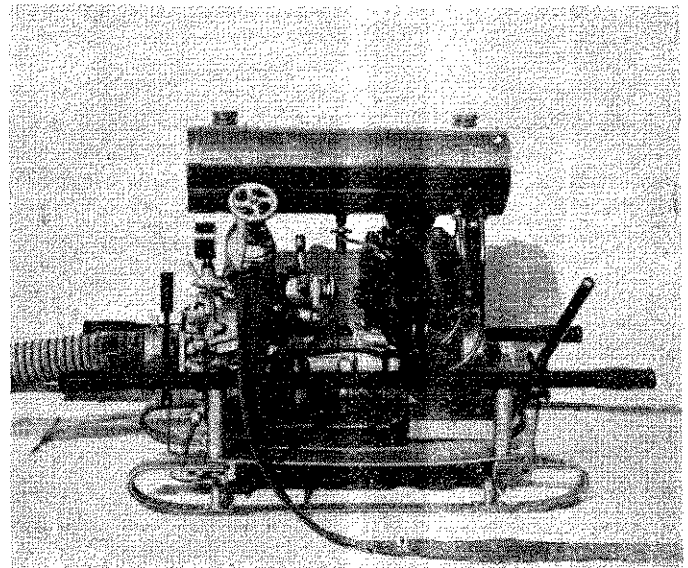
Magirus kismotorfecskendő (könnyűfém turbina, kétütemű motor, tisztavíz hűtés, könnyűfém gumitömítés nélküli szívótömlő csavar, 400 liter/8 atm. teljesítmény, tengelykapcsoló)
