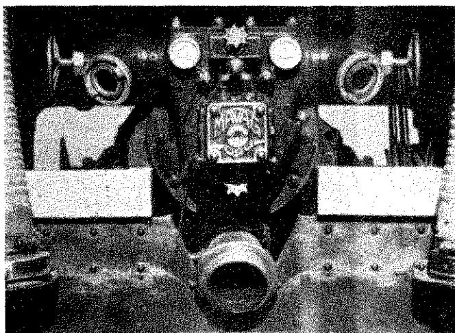
A hátul beépített „Turul” turbínaszivattyú
