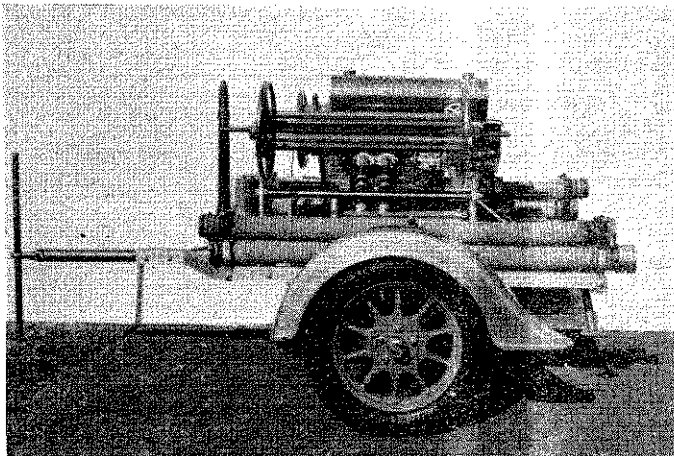
Magirus kismotorfecskendő
