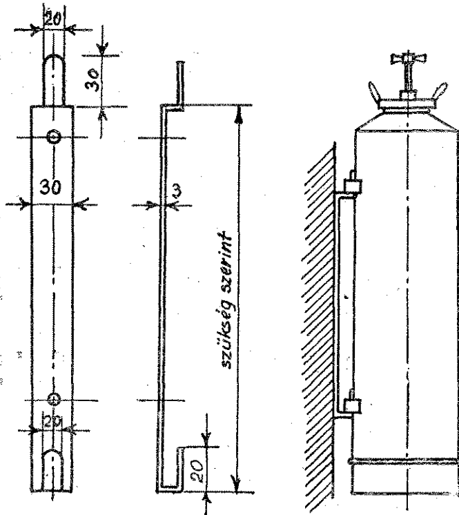
RÚGÓS FELFÜGGESZTŐ MOSz 1045 B — Javaslat Méretek mm-ben
