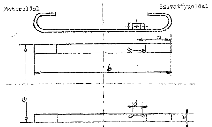
Kismotorfecskendők hordozóállványa
