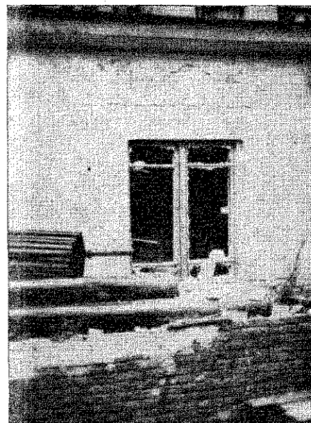
2. ábra. Az épület külső képe, a falon látható repedésnél a robbanás a vasbetonfödémét megemelte
