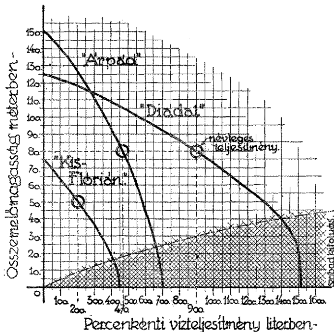
4. A három fecskendőteljesítmény diagramja
