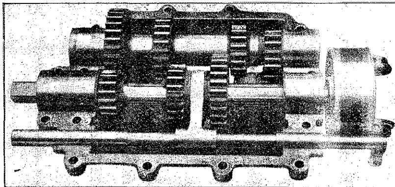
Egy benzín-automobil sebesség-váltója a különböző méretű s többféleféleképp kapcsolható fogaskerekekkel.
