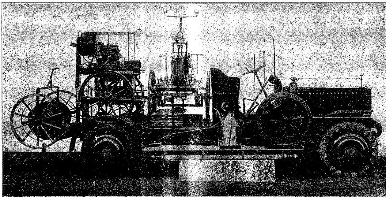
A konstantinápolyi tűzoltóság autofecskendője.
