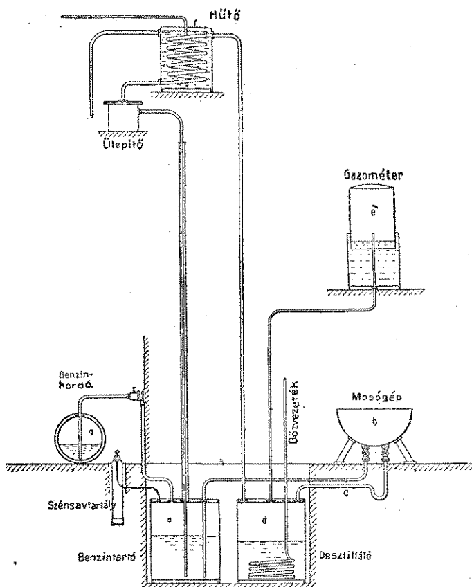
Az elhasznált benzín megtisztítására és újból való értékesítésére alkalmas berendezés szerkezete Martini-Hünecke szerint.
