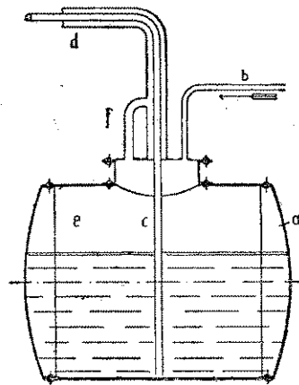
Benzintartály szerkezete.
