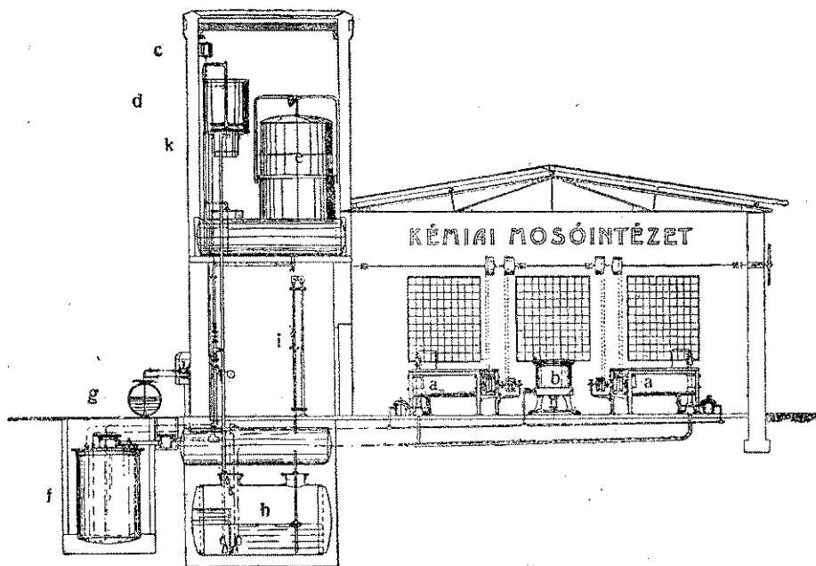
a mosógépek, b centrifuga, c vízcsap, d hűtő, e gázométer, f desztilláló, g benzintartó hordó, h benzintartály a földbe építve, i szintjelző készülék, k vizelválasztó.
