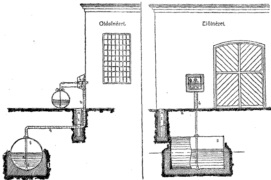
Gyúlékony folyadékoknak tűz és robbanás ellen biztos elhelyezése.
