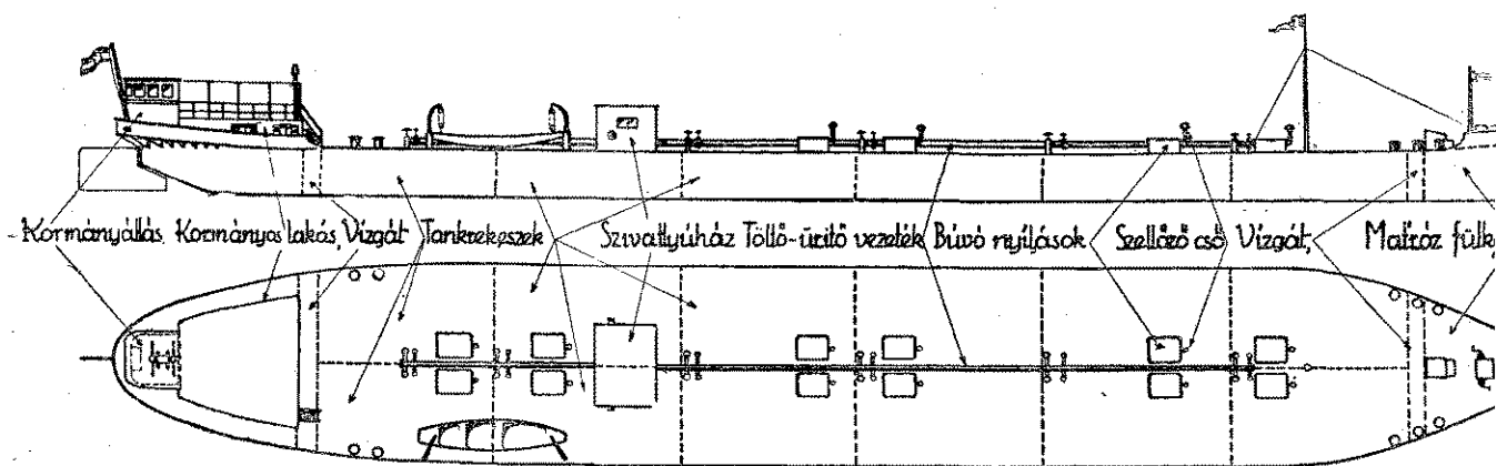
2. ábra. Tankuszályhajó elrendezési rajza
