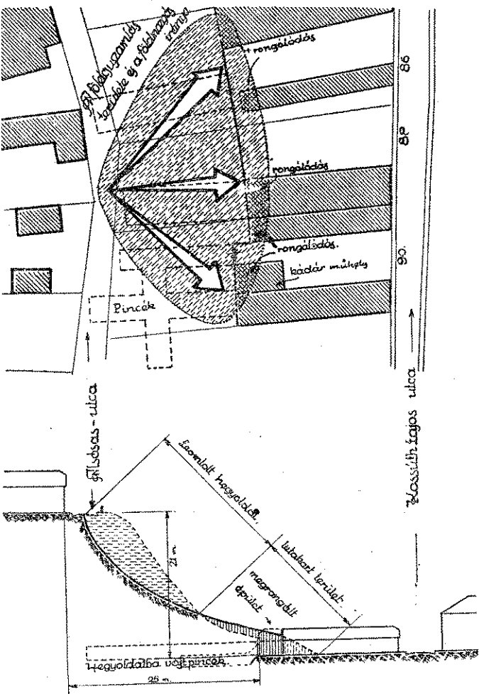
1. ábra. A földomlás helyszínrajza
