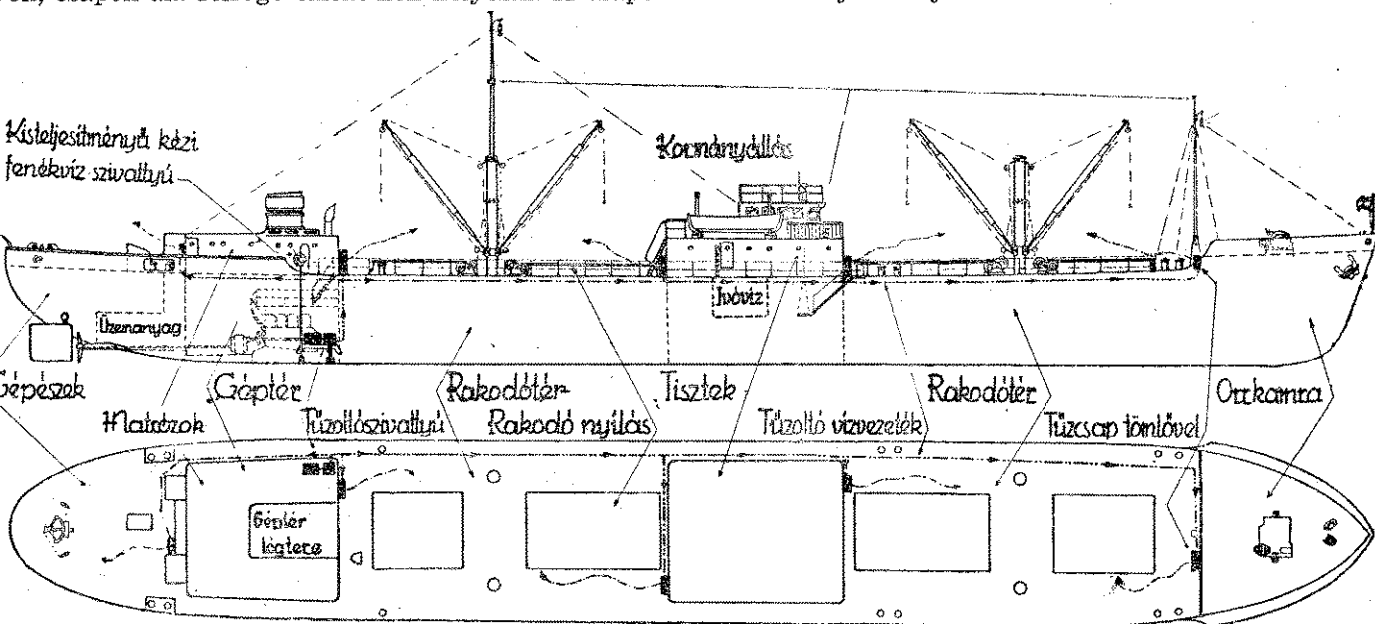
3. ábra. Egy Duna—tengerjáró hajó elrendezési rajza
