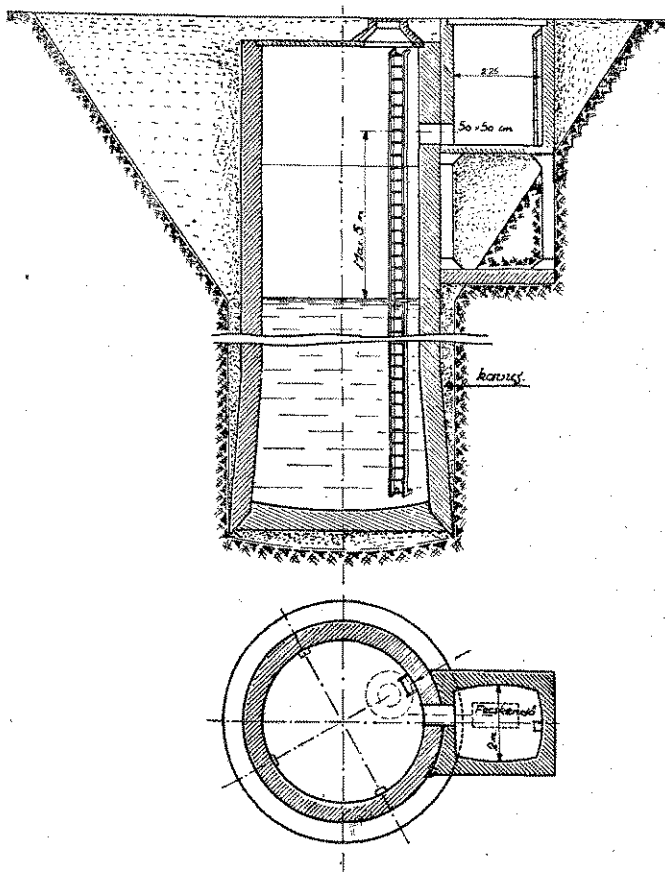
Tűzoltói célokra épült kút metszetrajza
