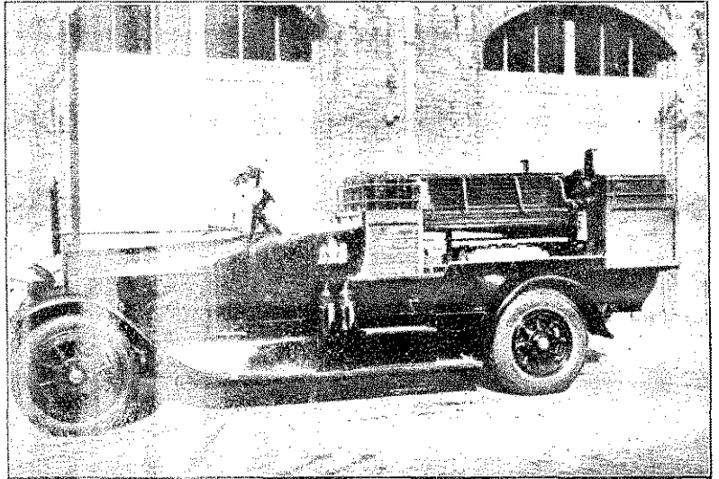
A haboltószer.
