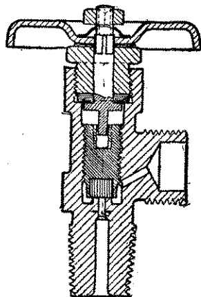
Gázszelep.
