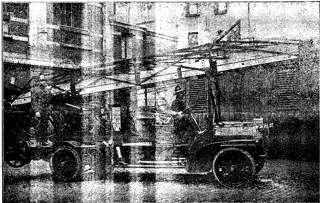
Magirus-féle autotolólétra villamos kihuzással. (Antwerpenben).
