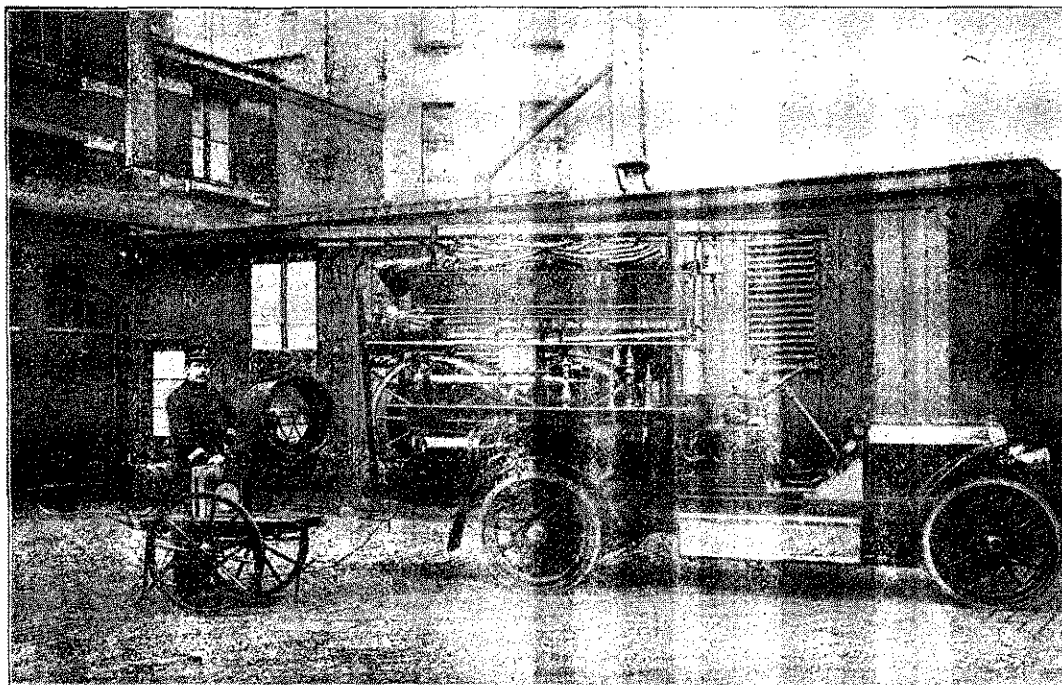
Az antwerpeni tűzoltóság szerkocsija és villamos fényvetője.
