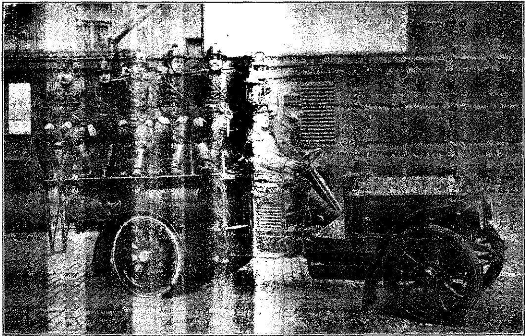
Az antwerpeni tűzoltóság auto-szerkocsija.
