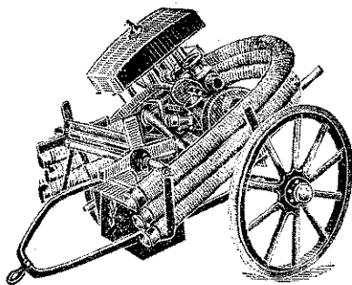
Mátrai cég motoros feeszkendője kétkerekű targoncára szerelve.
