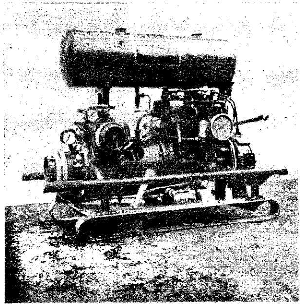
MAVAG gyártmányú 800 literes motorfecskendő
