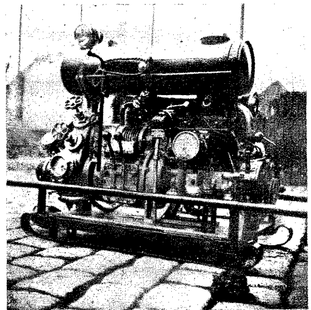
Flader — német — 800 literes víz és haboltó motorfecskendő
