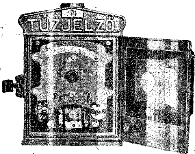
3. ábra. Tűzjelző állomás nyitott állapotban.
