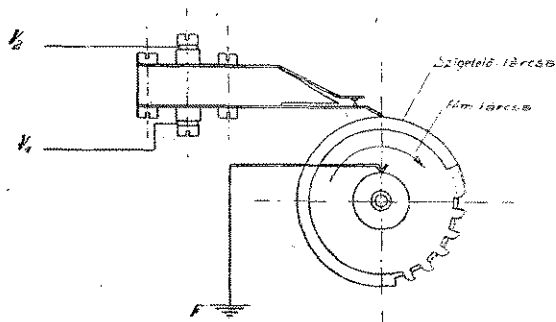
2. ábra. Tűzjelző állomás érintkezéseket adó szerkezete.
