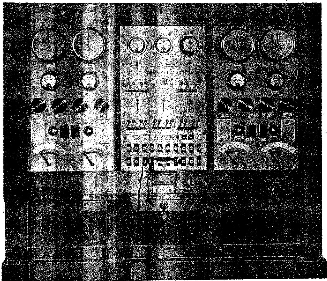
4. ábra. A tűzoltóórségen elhelyezett kapcsoló tábla.
