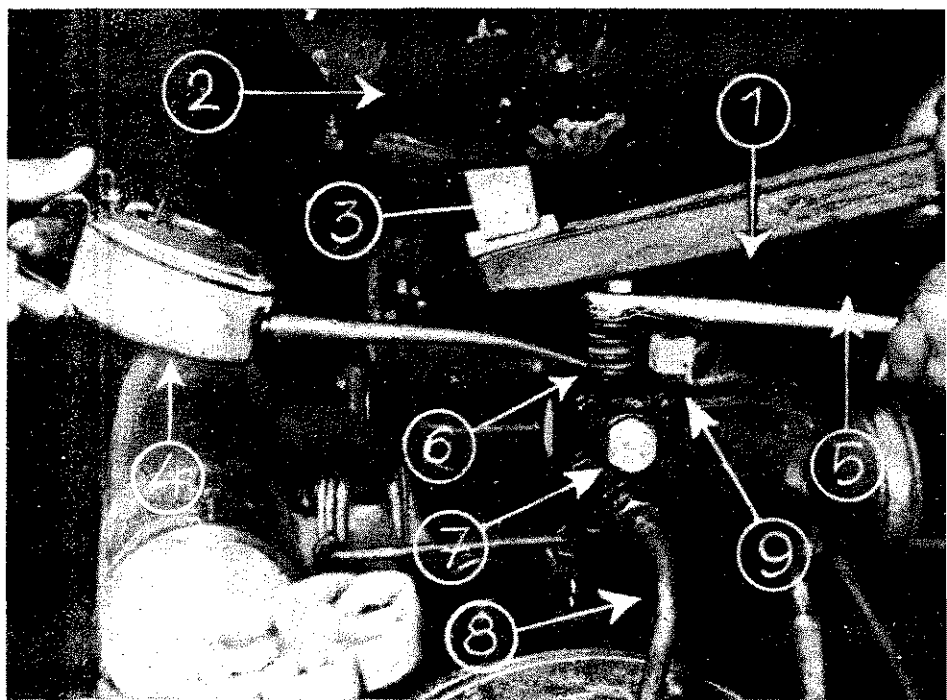
1. Kisebb vasrúd. — 2. Tartály. — 3. Fadarab. — 4. Olajozó kanna. — 5. Légtelenítőkar. — 6. Rúgó. — 7. Visszacsapószelep. — 8. Légtelenítőcső a szivattyúhoz. — 9. Szigetelő (rövidzárónál).
