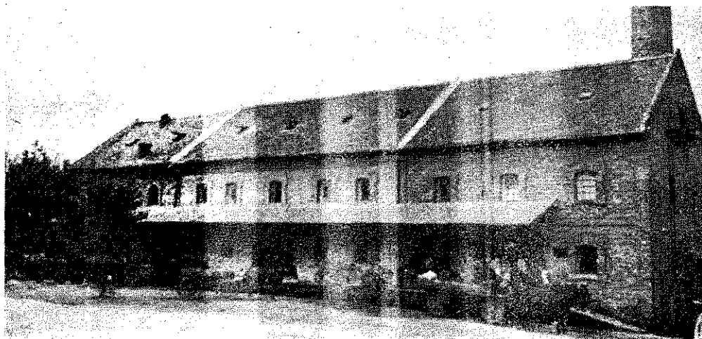
Közepes malom. — Jól láthatjuk az üzemszereket (koptató, malomrész, raktár) elválasztó tűzfalakat.
