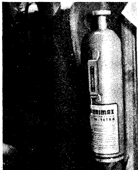
A gázzal oltó kézi tűzoltókészülék elhelyezése így helytelen, mert védőkupakkal nincs elzárva.
