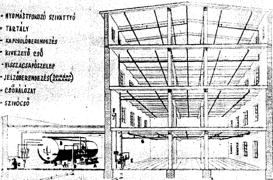
Nagy malomban felszerelt „sprinkler” készülék vázlatos rajza.
