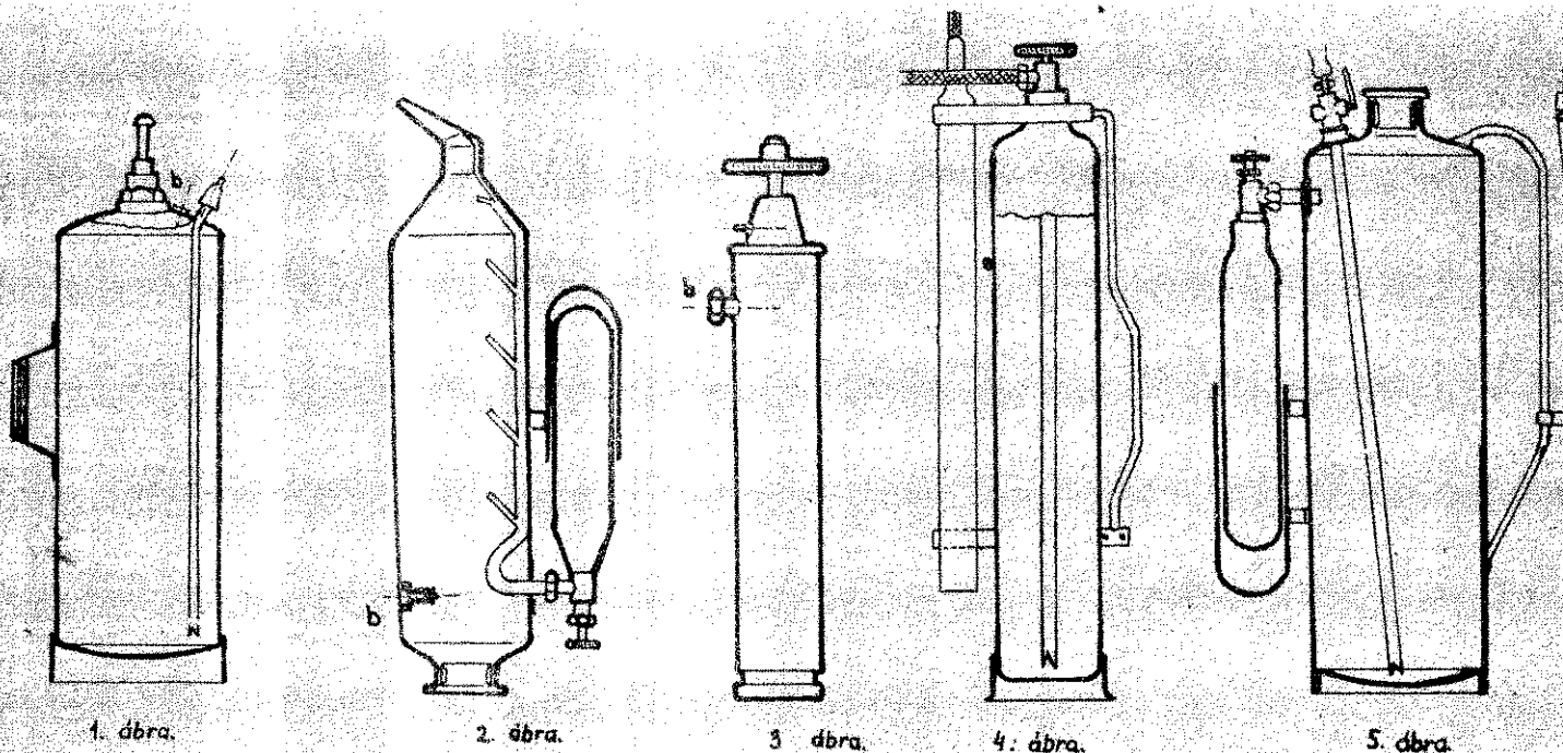
Különböző kézi tűzoltókészülékek.
