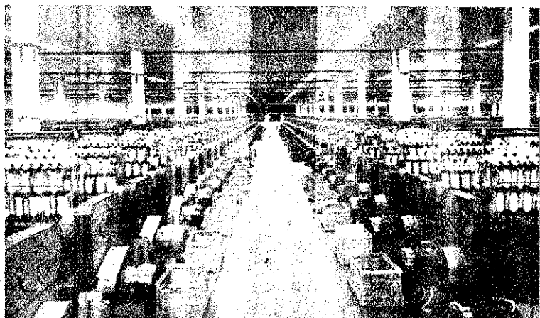
Korszerű fonóüzem, amely a megelőző tűzvédelem minden igényét kielégíti. A mennyezetén láthatók a „Sprinkler-rózsák” és a légtisztító berendezések.
