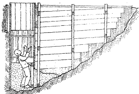
Mentés sekély gödörből
