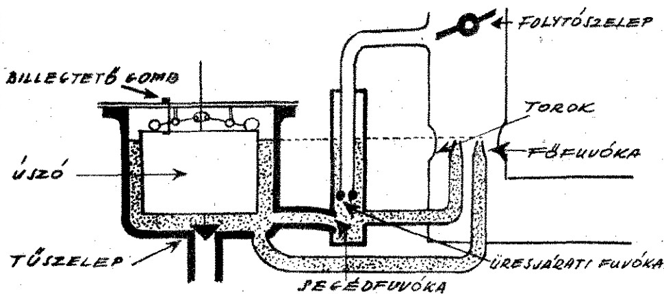
A porlasztó működése
