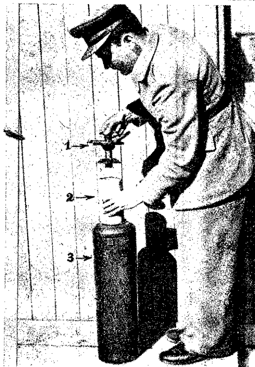
Vegyí habbal oltó tűzoltókészülék (1. Zárófejlél a lövőkével; 2. Savanyagot tartalmazó becső tartály; 3. Lúganyagot tartalmazó tartály.)
