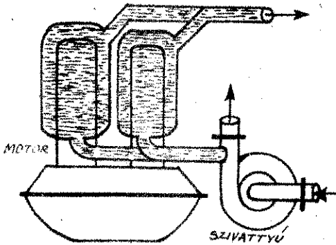
Atfolyó vízűtés
