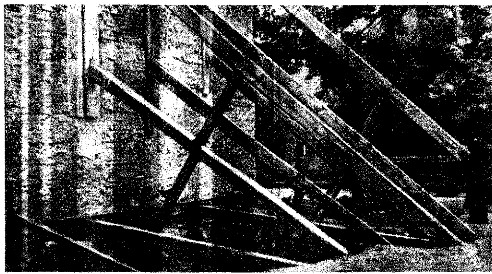
Megsérült fal kitámasztása
