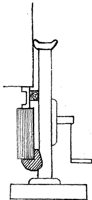
3. sz. ábra. Emelés fogásiéces emelő korméval
