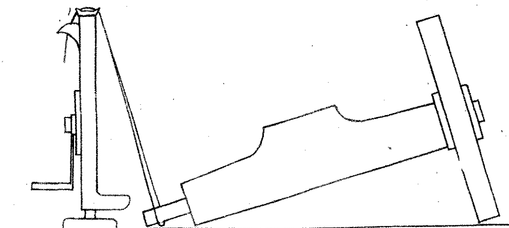
1. sz. ábra. Tengelycsap emelése fogasléces emelővel
