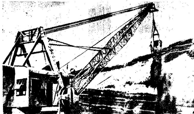
Gépesítés a szovjet bányákban. Egy „ES-1” típusú lépkedő exkavátor a szénpad megteremtésén dolgozik
