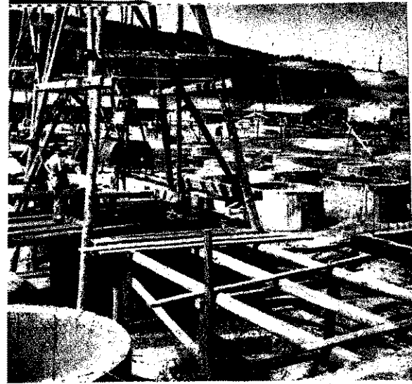
A Vegyiművek Beruházás Vállalat építkezése Kazincbarcikán. Népünk az új rendszerű, különlegesen nagyteherbírási alapozást mutatja be, amelynek lényege a gyűrűs és szakrényszerű megoldás.
