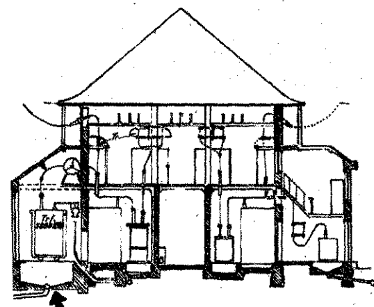
Transzformátor — állomás metszete olajgyújtómedencével és elfolyóval
