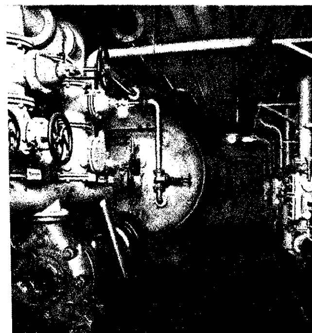
Sprinkler-állomás a víztartállyal
