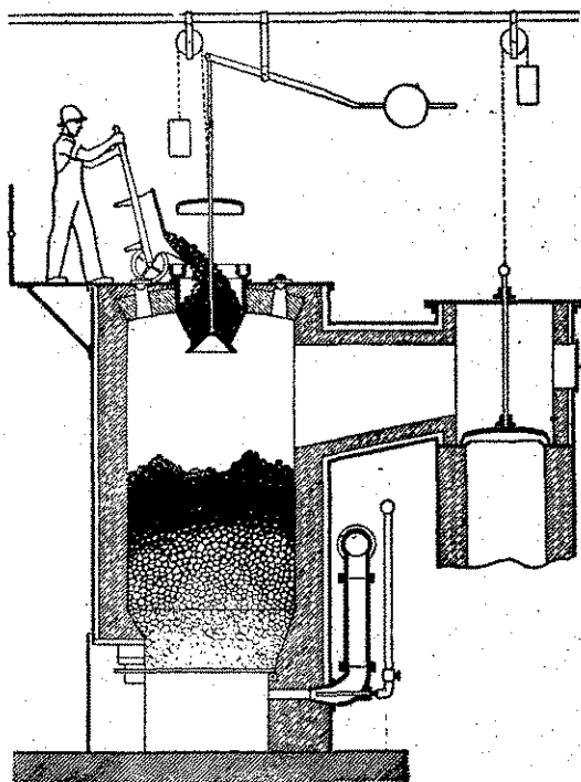
Generátor. Az akna alsó részében a rostélyra a jobboldali csövön bevezetett (esetleg vízgőzzel kevert) levegő segítségével a szén széndioxiddá ég el. Ez a felső réteg izzó szénével szénoxiddá alakul át.
