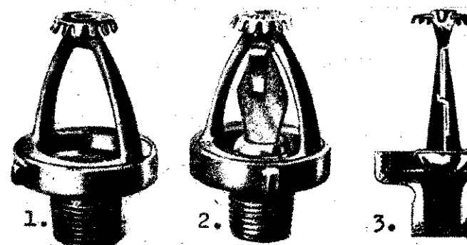
Sprinkler-rózsa. 1. Nyitva. 2. Zárva. 3. Működésben
