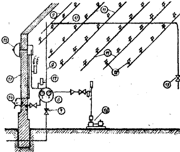
Szárazcsövű sprinkler-berendezés elvi rajza: 1. Magastartály, 2. sprinkler főnyomócső — 3. első víznyomócső — 4. vízszivattyú és denze — 5. vízoltattyú — 6. visszacsapó-szelep — 7. főtolattyú — 8. szárazcsövű főszelvény — 9. főelosztó cső — 10. elosztócső — 11. szárnyvezetékek — 12. sprinkler-rózsa — 13. légtelenítő-szelep — 14. víznyomócső — 15. riasztó gong — 16. villamos árammérő — 17. árammérő — 18. légtelenítő — 19. rózsa
