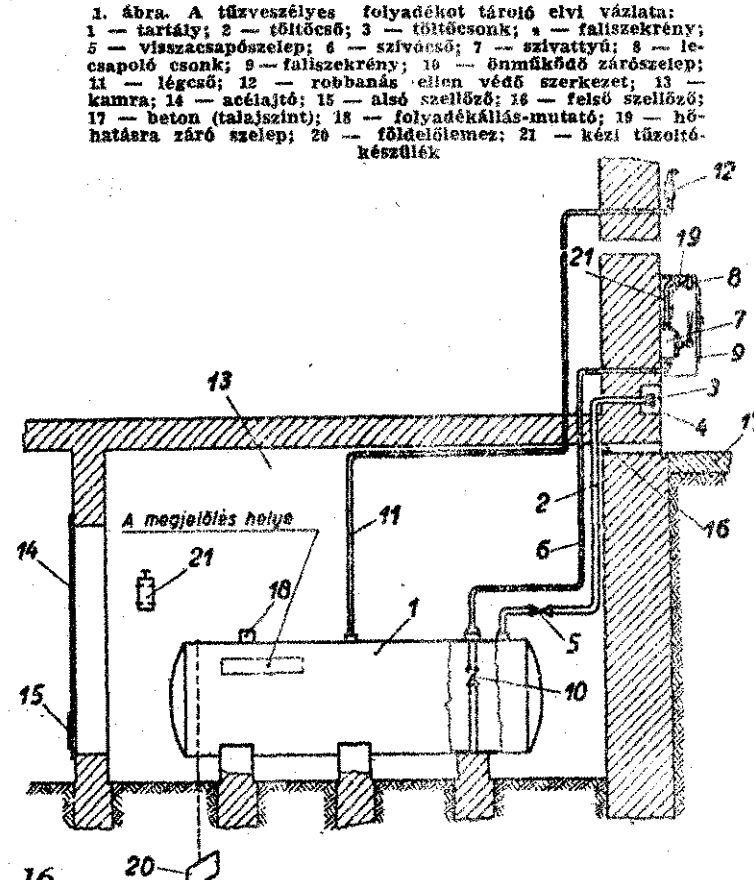
1. ábra. A tűzveszélyes folyadékok tároló elvi vázlata: 1 — tartály; 2 — töltőcső; 3 — töltőcső; 4 — faliszekrény; 5 — visszacsapószelep; 6 — szivócső; 7 — szivattyú; 8 — lecsapoló cső; 9 — faliszekrény; 10 — önműködő zárószelep; 11 — légső; 12 — robbanás ellen védő szerkezet; 13 — kamra; 14 — acélajtó; 15 — alsó szellőző; 16 — felső szellőző; 17 — beton (talajszint); 18 — folyadékállás-mutató; 19 — hőhatásra záró szelep; 20 — földelitemez; 21 — kézi tűzoltókészülék.
