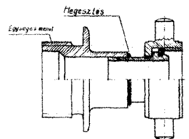
Áttéti darab a kézi működtetésű fecskendő szivócsontjára
