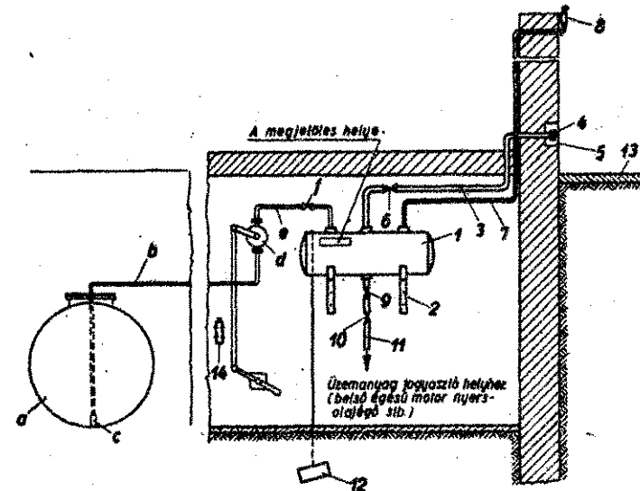
2. ábra. A tűzveszélyes folyadékok tároló napi üzemanyagtároló elvi vázlata: 1 — tartály; 2 — falitartók; 3 — töltőcső; 4 — töltőcső; 5 — faliszekrény; 6 — visszacsapószelep; 7 — légső; 8 — robbanás ellen védő szerkezet; 9 — hőhatásra záró szelep; 10 — elzáró szelep; 11 — üzemanyagcső; 12 — földelitemez; 13 — beton (talajszint); 14 — kézi tűzoltókészülék; a — tartály; b — szivócső; c — lábszelep; d — szivattyú; e — nyomócső; f — visszacsapószelep.
