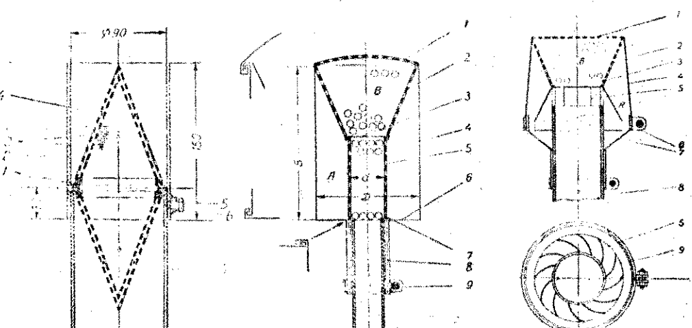
1. ábra 1 — préselt gyűrű; 2 — hegesztett cső; 3 — huzalháló; 4 — acélgyűrű; 5 — rögzítőcsavar; 6 — hegesztett alátét; 7 — a traktor kipuffogócsőve 2. ábra 1 — fedél; 2 — csónakakúp; 3 — a bevezető cső elzáró fedele; 4 — henger; 5 — bevezetőcső; 6 — hengerzáró fedéllemez; 7 — rögzítőcsavar; 8 — felerősítő cső; 9 — kegyel 3. ábra 1 — fedél; 2 csónakakúp; 3 — fenékrész; 4 — szikrafogó teste; 5 — terelőlapátok; 6 — gyújtó oldalifalak; 7 — gyújtótálcák; 8 — Diesel-motor kipuffogócsőve; 9 — csatornák
