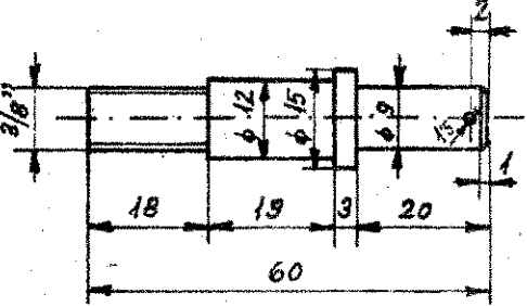
250-es motorkerékpárok berúgó félfogaskerék ütközőjének javítása
