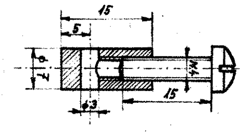
Bowden-vezetékek belső huzalvégének javítása
