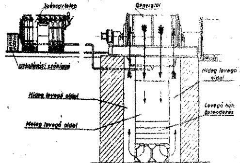
A rendszer vízmentes beépített szénsavoltó berendezés működési vázlatja
