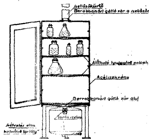
A tűzveszélyes folyadékok tárolására szolgáló robbanásálló szekrény vázlatos rajza
