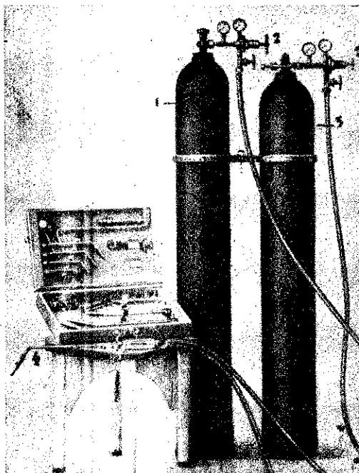
Autogénhegesztő berendezés: 1. oxigéntartály; 2. nyomásosökentő szelepek; 3. dissoungáz-tartály; 4. hegesztőpisztoly
