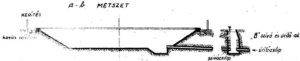
A szabályosan épített víztároló medence keresztmetszet rajza
