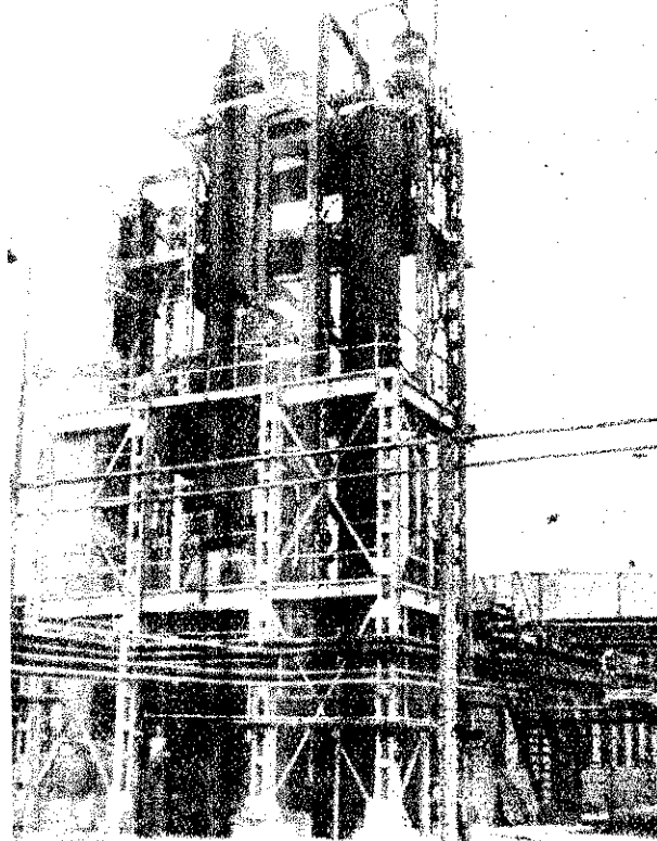
A lepárló — az extrakció legfontosabb he- lye — kiválasztja a kész terméket és az üzembe visszajuttatja a butilacetátot
