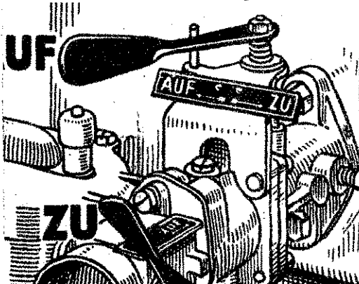
Kétkaros Solex karburátor hideg indítási helyzetben
