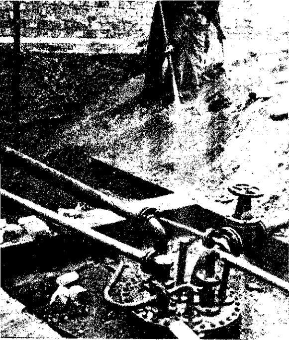
A szabvány szerint megépített földalatti tárolóban biztosítják a desztilláló fűtőanyagát, a gázolajat
