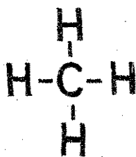
A metán szerkezeti képlete
