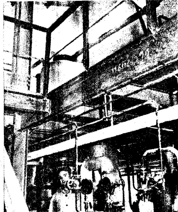
A desztilláló falai teglából, földem- és tető- szerkezete vasból, illetőleg lemezből készül
