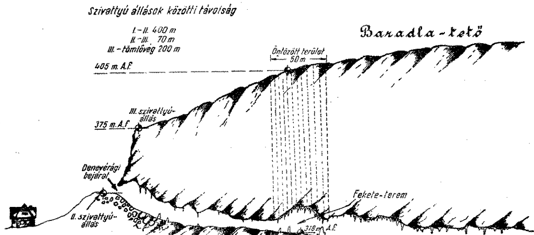
Az aggteleki árasztás vázlata
