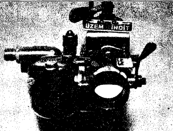
Kétkaros Solex karburátor — helytelen magyar felirattal — indítási helyzetben
