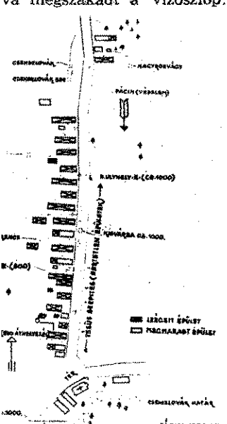
Helyszínrajz
