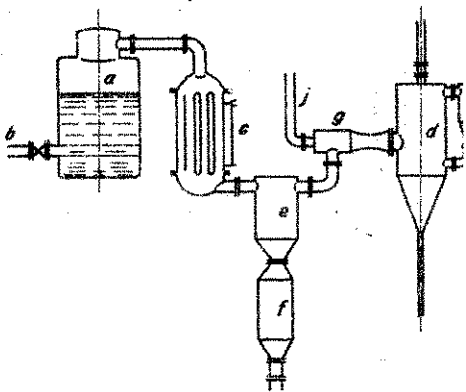
A Lurgi-féle zsírsavdesztilláló berendezés vázlata
