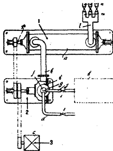
Schroeder van Deurs habfejlesztő felszerelése
