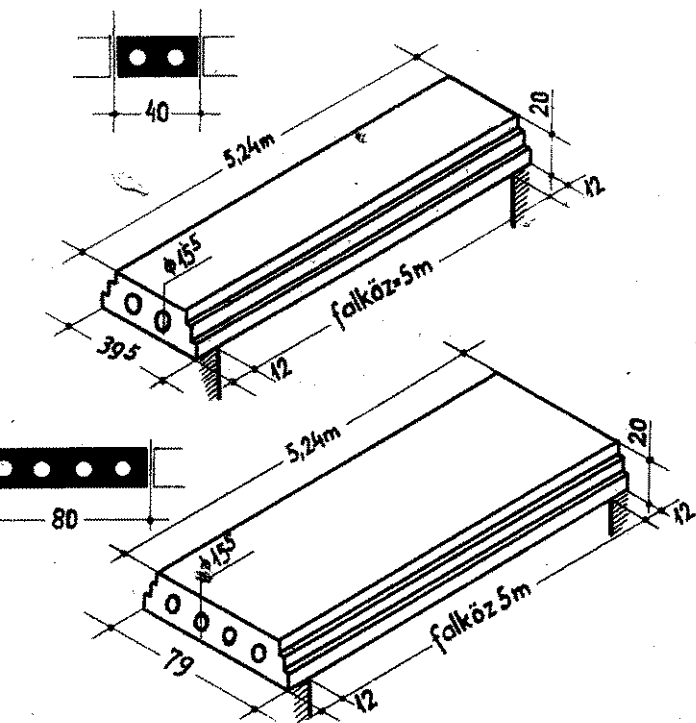
SZIM-KAR födémpanel
