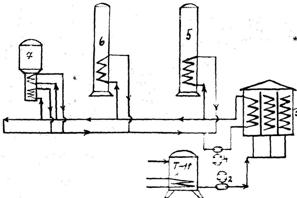
Csőkemencés fűtőrendszer
