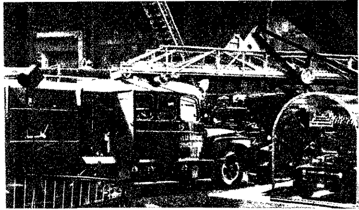
A brüsszeli világkiállításon tűzoltó szerek és felszerelés mutatására is sor került. Felső képünk a kiállított szerencsoportját, alsó képünk pedig az ostendei tűzoltóság na kisnyomású kombinált szivattyúval ellátott tartályos műfecskeendőjét ábrázolja
