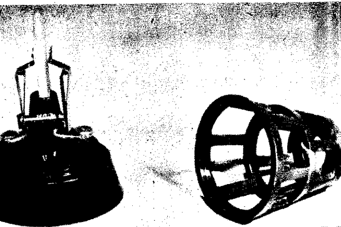
Az új tűzjelző hőészlelő prototípusa
