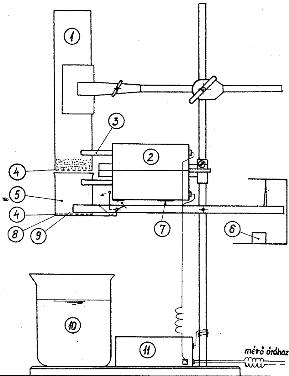
Porszóró készülék porlekötési vizsgálatokhoz
