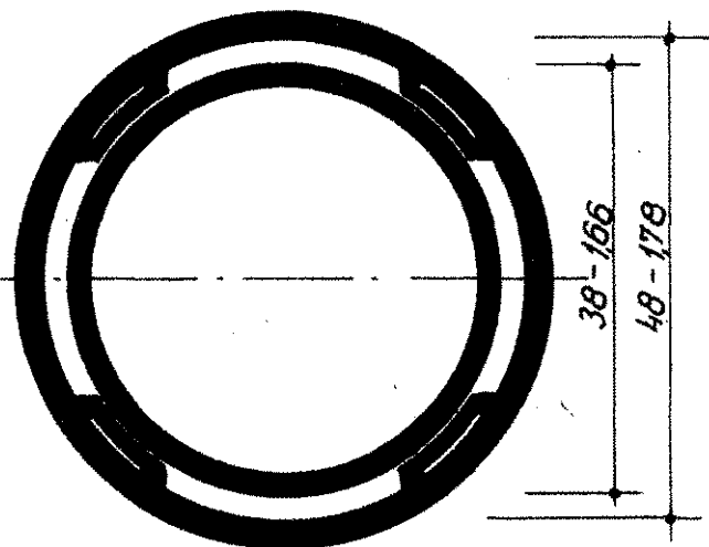
Központi fűtési kéményelemek
