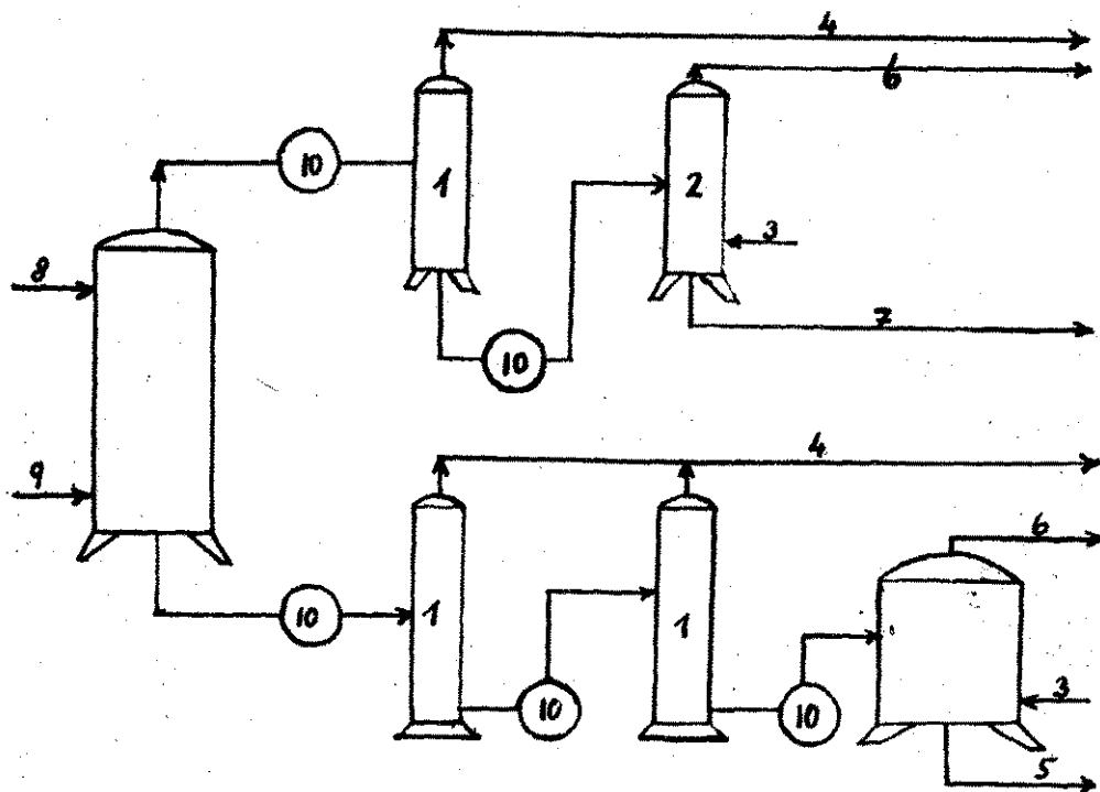
Furfurolos (oldószér) visszanyerő vázlata:
