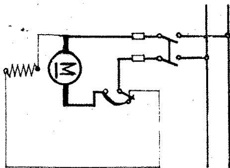
Egyenáramú, mellékáramkörű motor
