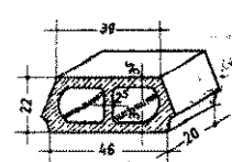
Födém beléstegek
