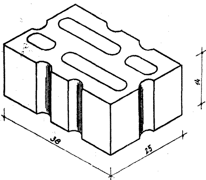
Falazó salakbeton blokk
