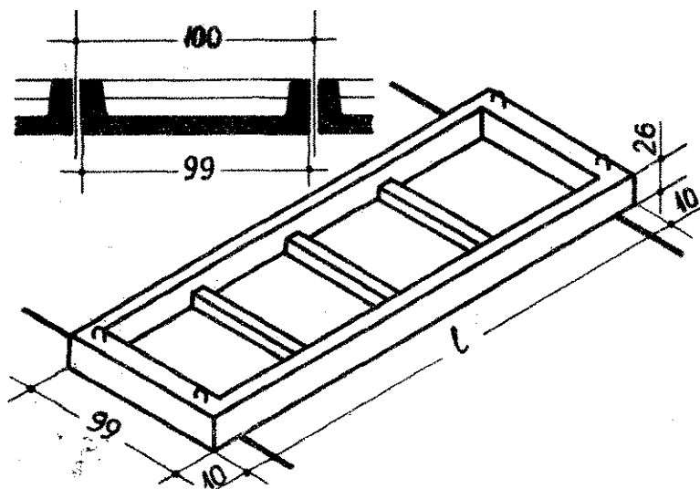
Felül bordás födémpanel
