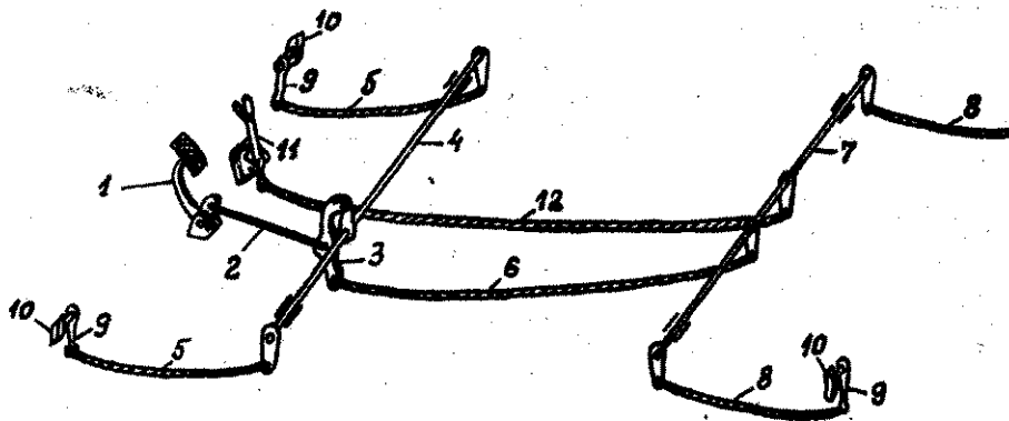
2. ábra. Mechanikus fék vázlata:
