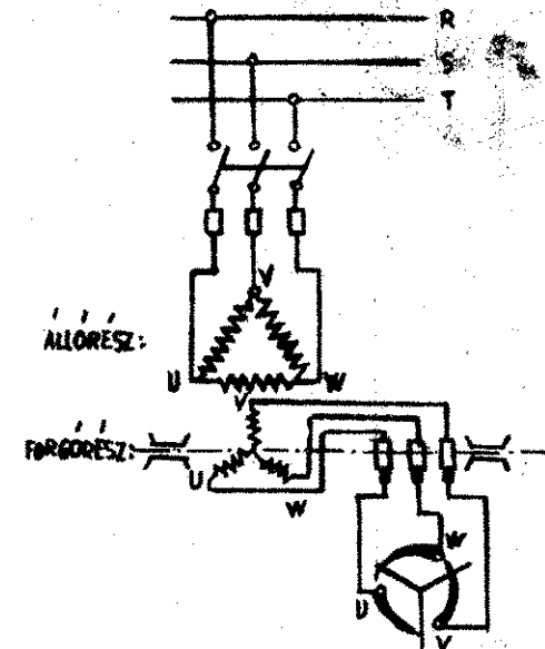
Csúszógyűrűs indukciós motor
