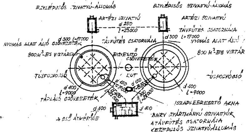
A vízvezeték-hálózatot tápláló állomásrendszer egyik lehetséges
