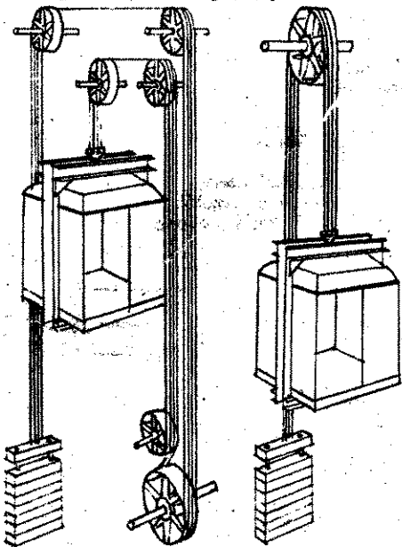
Alsó- és felsőgépes felvonó
