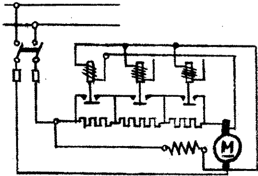
Kapcsolótekeres-önindító — egyfázisú motornál
