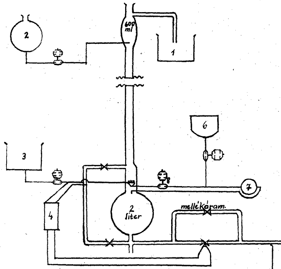
Olajfinomító berendezés laboratóriumi ellenőrzéshez:
