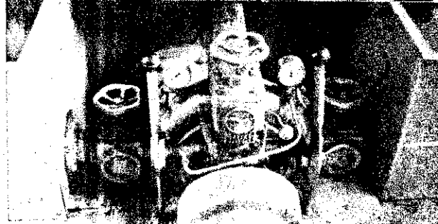
Az ülés alatt elhelyezett szivattyú
